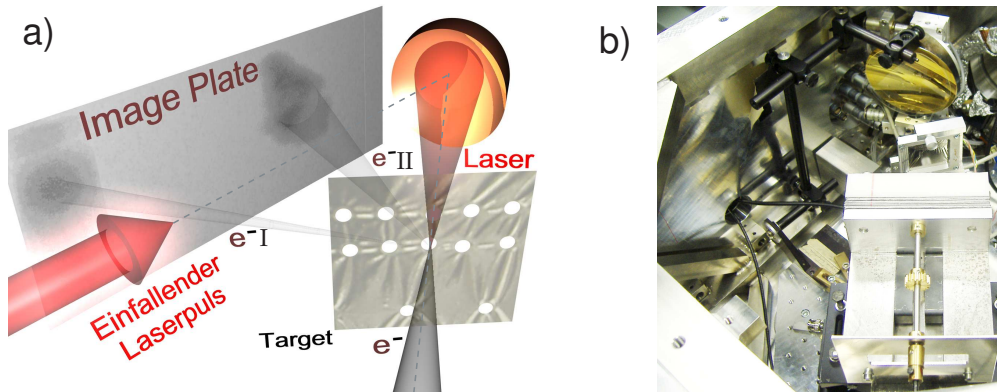
Abbildung 23: Versuchsaufbau. a) Computer-Reproduktion des Versuchsaufbaus mit Projektion der Originalrohdaten des Elektronensignals auf der Image Plate. Der einfallende Laserpuls wird von der Parabel reflektiert und fokussiert, trifft auf das Target und ruft dort Emission von Elektronen in verschiedene Richtungen hervor, die großflächig mit Image Plates detektiert wurden. b) Foto des Versuchsaufbaus aus demselben Winkel, hier ist die Image Plate von einem Al-Schutzblech geschützt und es ist zusätzlich noch das Elektronenspektrometer zur Messung der Elektronen in Vorwärtsrichtung sichtbar.
