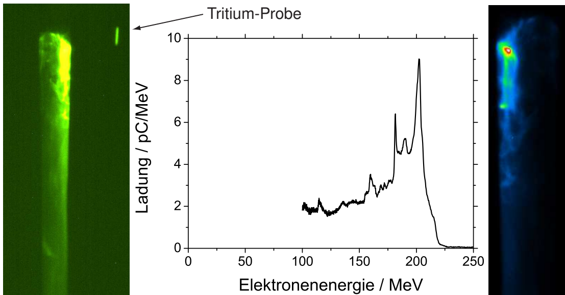
Abbildung 95: Rohdaten auf dem Lanex-Schirm und ausgewertetes Elektronenspektrum. Links: Rohsignal eines Elektronenschusses auf dem Lanex-Schirm in einer Darstellung, in der man das im Vergleich zum Elektronensignal schwach leuchtende Tritium-Röhrchen erkennt. Rechts: derselbe Schuss auf dem Lanex-Schirm mit Falschfarbendarstellung, aus dem der monoenergetische Peak deutlich hervorgeht. Mitte: ausgewertetes Spektrum mit einem signifikanten peak bei etwa 200 MeV.
