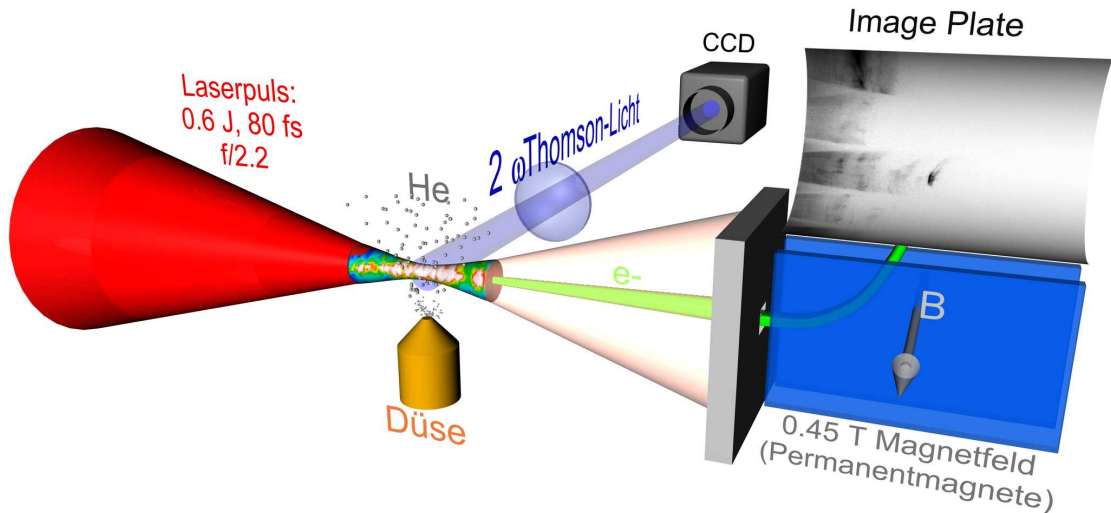
Abbildung 64: Versuchsaufbau zur Erzeugung und Detektion monochromatischer, relativistischer Elektronen über Laser-Plasma-Wechselwirkung. Der fokussierte Laserpuls erzeugt im Gas-Jet einen Plasmakanal, der über Thomsonstreuung beobachtet werden kann. Die beschleunigten Elektronen können mit Hilfe eines Permanentmagnet-Elektronenspektrometers und Image Plates detektiert werden. Nicht abgebildet sind der Beam Viewer, das Spektrometer zur Detektion des transmittierten Laserlichts und die Ionisationskammer (veröffentlicht in [4], Figure reprint permission from Physical Review Letters ).
