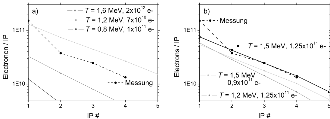
Abbildung 49: Resultate des iterativen Stack-Auswerteverfahrens. b) zeigt, dass mit der Methode sowohl die Gesamtzahl als auch die Temperatur des gemessenen Strahls sehr exakt rekonstruiert werden kann.
