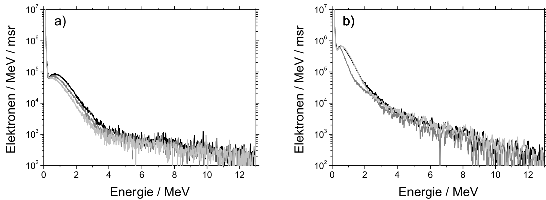
Abbildung 36: Gemessene Elektronenspektren in Vorwärtsrichtung bei einer Intensität von etwa I_L \approx 2 \cdot 10^{19} \text{ W/cm}^2 und a) 5 \mu\text{m} Titanfolie, b) 25 \mu\text{m} Titanfolie als Target.
