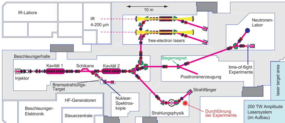
Abbildung 98: Aufbau des ELBE-Beschleunigers am FZD und Implementierung des 200 TW-Lasersystems. Die Kalibrationsexperimente fanden im Strahlungsphysik-Cave statt. Der genaue Ort ist mit dem roten Stern markiert (Abbildung auf Grundlage einer vom ELBE-Team zur Verfügung gestellten Zeichnung [289]).
