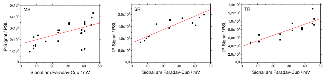
Abbildung 99: Kreuzkalibration dreier verschiedener IP-Typen mit einem Faraday-Cup an ELBE. Links: MS-Typ, Mitte: SR-Typ, Rechts: TR-Typ.
