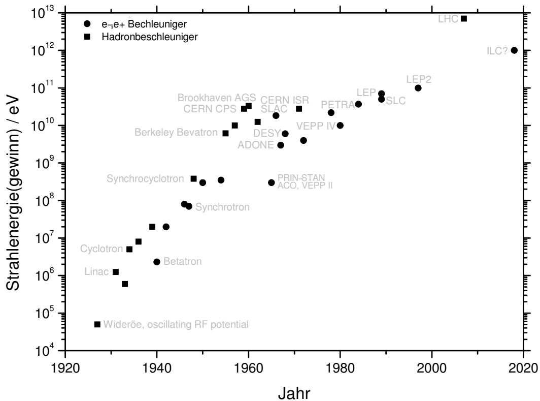
Abbildung 8: Livingston-Plot. Es sind die jeweils maximal erreichbaren Energien sowohl für Elektronen- und Positronenbeschleuniger angegeben als auch die für die Beschleunigung von Protonen und anderen Hadronen.
