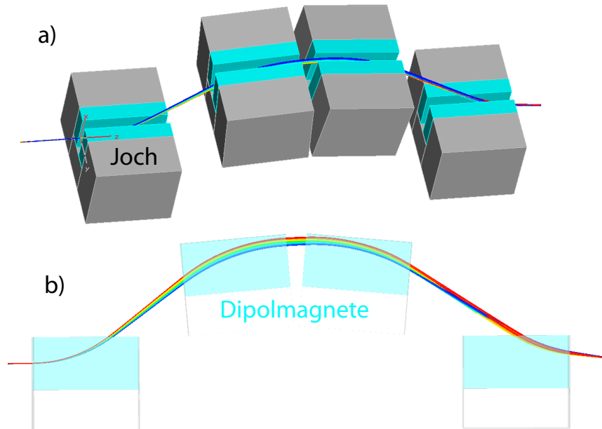
Abbildung 12: Zeitlichen Komprimierung eines gepulsten Elektronenpulses beim Durchlaufen einer magnetischen Schikane. a) 3D-Ansicht, in der man die vier Dipolmagnete erkennt. b) Seitansicht. Der Puls kommt von links, die blauen, hochenergetischen Anteile legen eine größere Distanz als die roten, niederenergetischen Anteile zurück.
