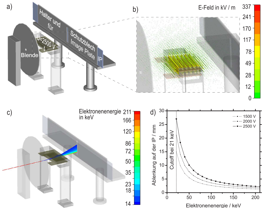
Abbildung 17: Elektrisches Elektronenspektrometer. a) Aufbau. Nach Passieren der Blende wird der von links kommende Elektronenstrahl in einer Hochspannung zwischen Anoden- und Kathodenplatte abgelenkt und wird dann pro Schuss auf einem schmalen Streifen der beweglichen Image Plate aufgenommen. b) Simulation des elektrischen Feldes zwischen den Ablenkplatten. c) Simulierte Trajektorien der Elektronen mit Energien bis ca. 200 keV. d) Aus der Simulation erhaltene Kalibration für die Ablenkung der Elektronen.
