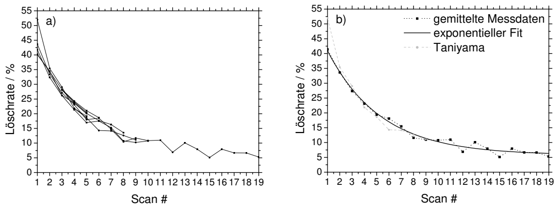
Abbildung 41: a) Relative Löschraten des Signals auf der IP mit der Anzahl der Scans. b) Gemittelte Löschraten, exponentieller Fit und Vergleich zu Daten aus [151] (nicht zeitbereinigt).
