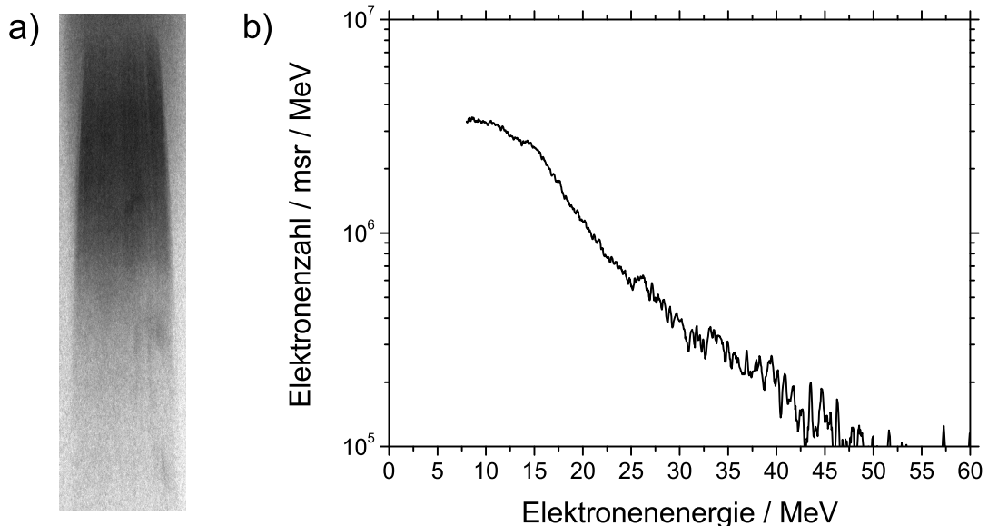
Abbildung 71: Gemessenes Elektronenspektrum. a) Rohdaten auf der IP und b) ausgewertetes, typisches Spektrum mit exponentieller Energieverteilung. Die Temperatur der Verteilung beträgt hier T_{\text{eff}} \approx 8 \text{ MeV} .
