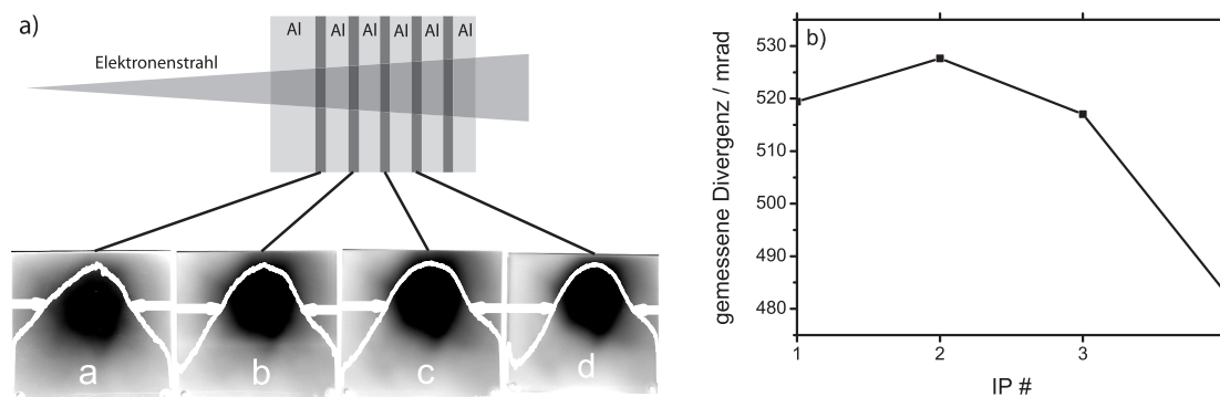
Abbildung 52: Auswertung der Divergenz des Elektronenstrahls auf den einzelnen IPs. a) Lineouts der Rohdaten, b) Plot der auf den hintereinander positionierten Stack-IPs.
