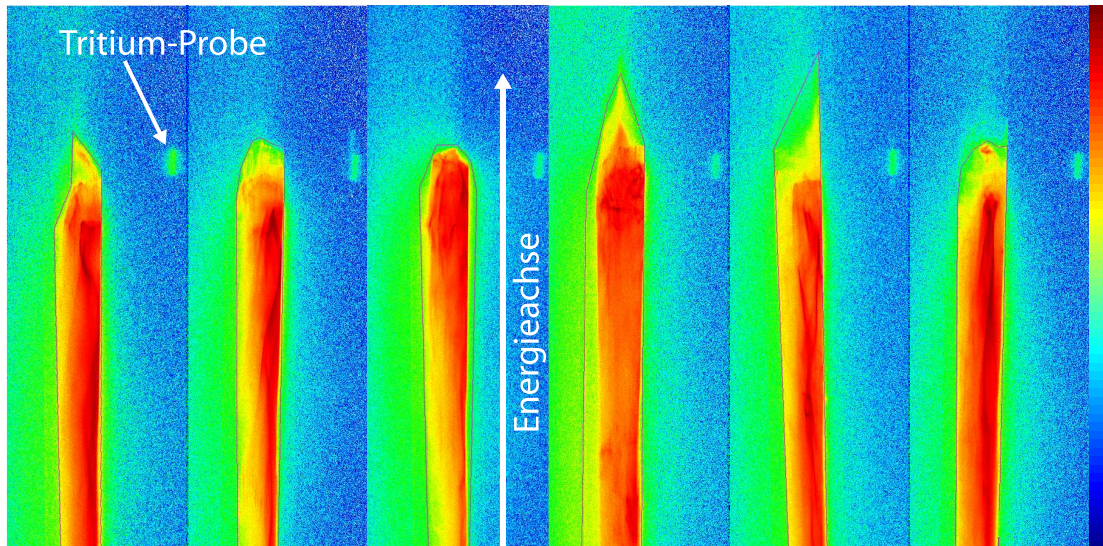
Abbildung 94: Image Plate-Bilder einzelner Elektronenbunches in der Detektionsebene hinter dem Spektrometer. Die Energieachse verläuft von unten nach oben. Die hier erreichten Maximalenergien liegen alle bei etwa 200 MeV.
