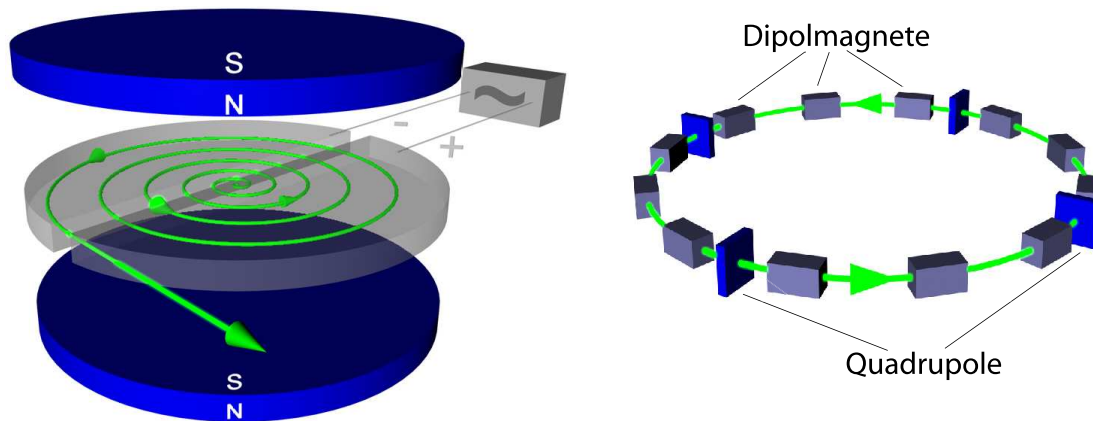
Abbildung 9: Schemata von Cyclotron (links) und Synchrotron (rechts).
