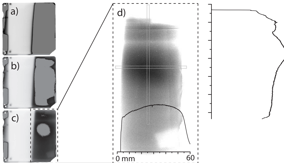
Abbildung 25: Rohdaten der wiederholten Scans der Targetparallelen-IP. In den Scans a)-c) ist eine einfarbig grau eingefärbte, kleiner werdende Region zu erkennen, die dem Scanvorgang gegenüber „überbelichtet“ ist. Mit dem vierten Scan d) kann schließlich das verbleibende Restsignal auf der IP aufgelöst und ausgewertet werden. Es ergibt sich für den Peak eine (horizontale) Halbwertsbreite von etwa 53 mm entsprechend einer Divergenz von etwa 209 mrad.
