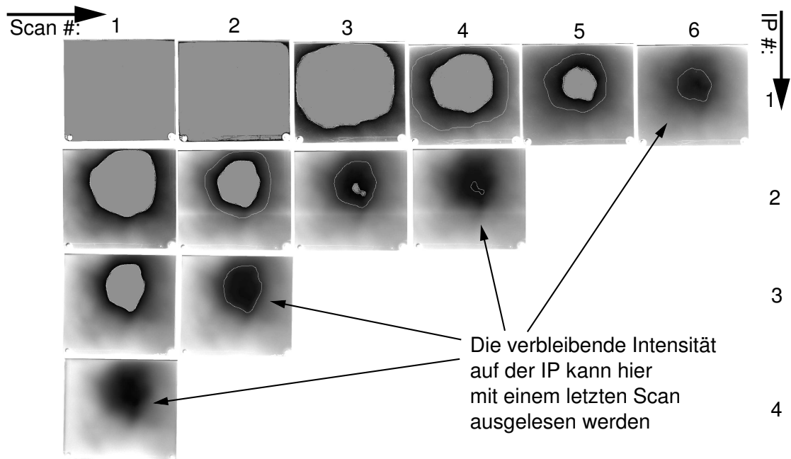
Abbildung 43: Rohdaten auf den Image Plates aus dem Stack. Von links nach rechts nimmt die Scananzahl zu, von oben nach unten sind die vier IPs je nach Position im Stack (von vorne nach hinten) angeordnet. Während für die erste, vordere IP, insgesamt sechs Scans notwendig sind, um die gesamte Signalintensität auf der IP auszulesen, ist die Intensität auf der letzten IP so gering, dass ein einzelner Scan ausreicht.
