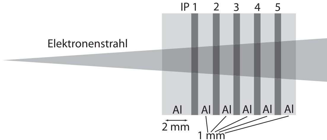
Abbildung 42: Experimenteller Aufbau für die IP-Stack-Messungen. Hinter einer Frontplatte aus 2 mm starkem Aluminium folgen alternierend IPs und weitere 1 mm dicke Al-Filter.
