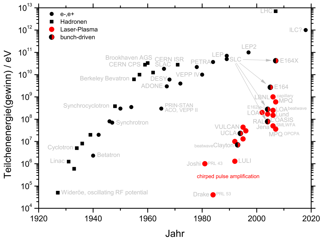
Abbildung 102: Um Laser-Plasma-Beschleuniger erweiterter Livingston-Plot. In rot ist eine Auswahl von Laser-Plasma-Beschleunigerexperimente eingetragen, inklusive der SMLWFA in Jena, der LWFA mit dem OPCPA am MPQ, und der Kapillar-Experimente mit dem ATLAS am MPQ. In schwarz/rot sind Experimente zur bunch-driven Wakefield acceleration eingetragen, die fast alle am SLAC stattgefunden haben.
