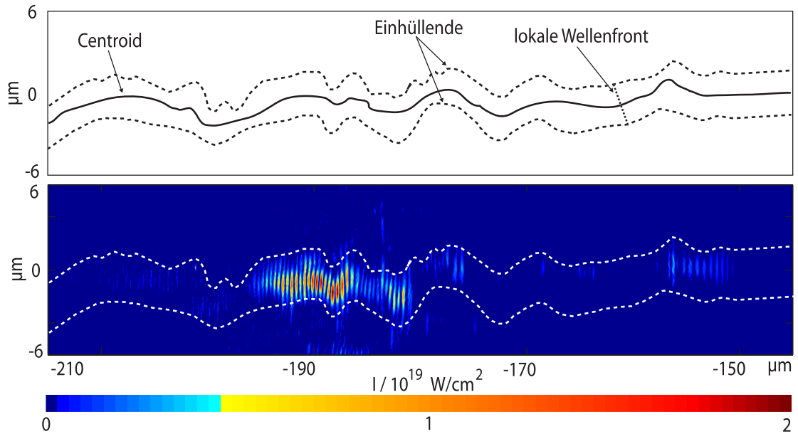
Abbildung 82: Hosing des Laserpulses. Die Vergrößerung aus Abbildung 80 f) verdeutlicht dieses Phänomen, dessen Stärke mit höherer Dichte ansteigt, guiding behindern und zu schlechterem pointing und schlechterer Divergenz führen kann.
