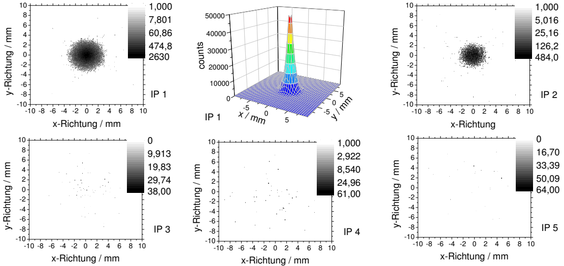
Abbildung 53: Monte-Carlo-Simulationen mit GEANT4. Streuung von Elektronen mit einer Energie von E = 2 MeV im IP-Stack. Die einzelnen Bilder sind zwei- beziehungsweise dreidimensionale, farbkodierte Visualisierungen der Anzahl der Events in den sensitiven Schichten der einzelnen IPs.
