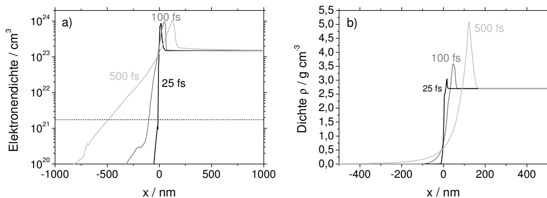
Abbildung 15: Hydrodynamische 1D-Simulationen mit MULTI-FS für einen relativistischen Laserpuls mit einer Spitzenintensität von 10^{18} W/cm 2 . Man erkennt sowohl im Elektronenbild (a) als auch im Dichtebild (b) in den Festkörper hineinlaufende Schocks.
