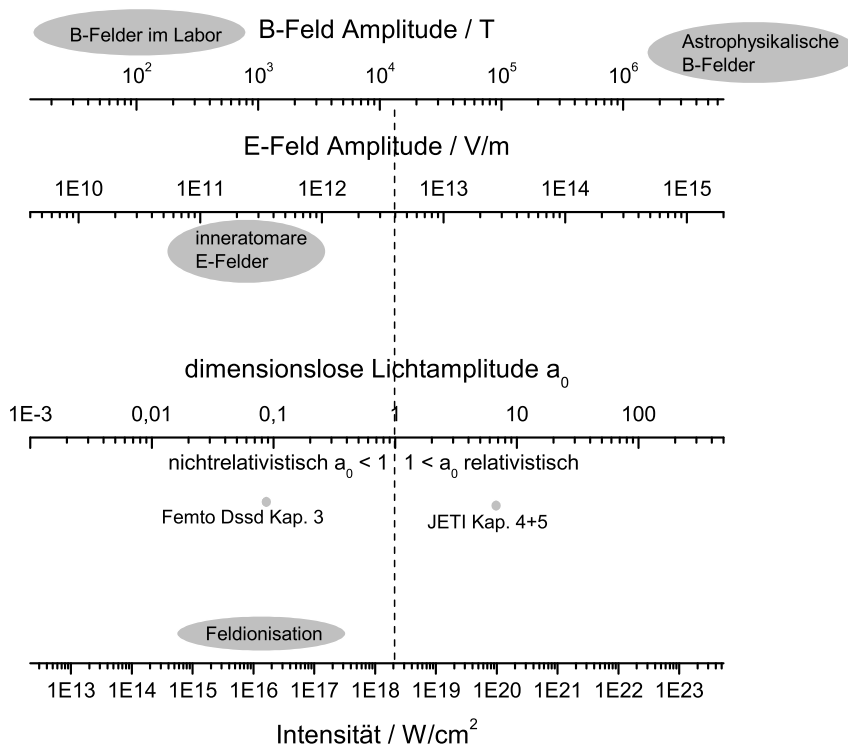
Abbildung 7: Graphische Darstellung des Zusammenhangs zwischen Laserpulsintensität, sowie der sich dadurch ergebenden Lichtamplitude a_0 und den dazugehörigen maximalen elektrischen und magnetischen Feldern. Der Übergang vom nicht-relativistischen zum relativistischen Bereich ist durch a_0 = 1 gegeben.
