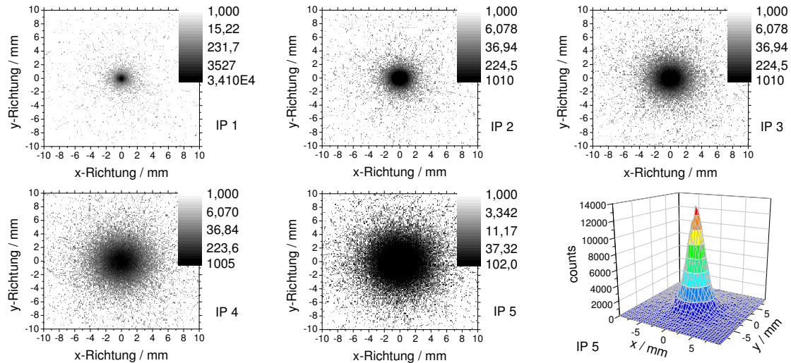
Abbildung 54: Monte-Carlo-Simulationen mit GEANT4. Streuung von Elektronen mit einer Energie von E = 10 MeV im IP-Stack.
