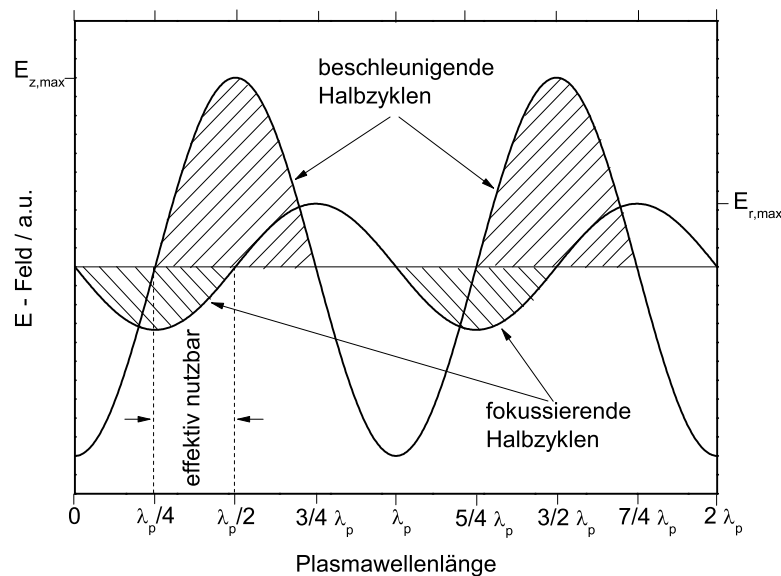
Abbildung 60: Schemazeichnung der Überlagerung von beschleunigender und bremsender sowie fokussierender und defokussierender Phase in einer dreidimensionalen Plasmawelle. Nur ein Bereich mit einer Breite von \lambda_p/4 kann sinnvoll zur Teilchenbeschleunigung benutzt werden.
