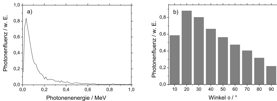
Abbildung 47: MULASSIS-Ergebnisse für die entstehende Bremsstrahlung im Stack. a) Spektrum der durch den Einfall eines exponentiellen Elektronenstrahls in der stirnseitigen Al-Blende vor der ersten IP erzeugten Bremsstrahlung, b) Winkelverteilung dieser Bremsstrahlung.
