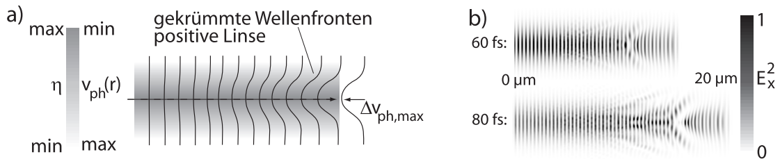
Abbildung 62: a) Schematische Veranschaulichung der Selbstfokussierung. b) 2D-PIC-Simulation mit PSC zur relativistischen Selbstfokussierung für einen Laserpuls der Dauer 80 fs, für eine Intensität von I = 10^{19} \text{ W/cm}^2 , eine Breite (FWHM) von 5 \mu\text{m} und eine Gasdichte von n_e = 10^{20} \text{ cm}^{-3} . Es ist jeweils das Quadrat des E -Feldes des Laserpulses in der Polarisationssebene gezeigt. Der obere Schnappschuss wurde etwa 60 fs nach Eintritt in die Simulationsbox von links aufgenommen, der untere 20 fs später. Die relativistische Selbstfokussierung nimmt mit zunehmender Propagationsdistanz deutlich zu.
