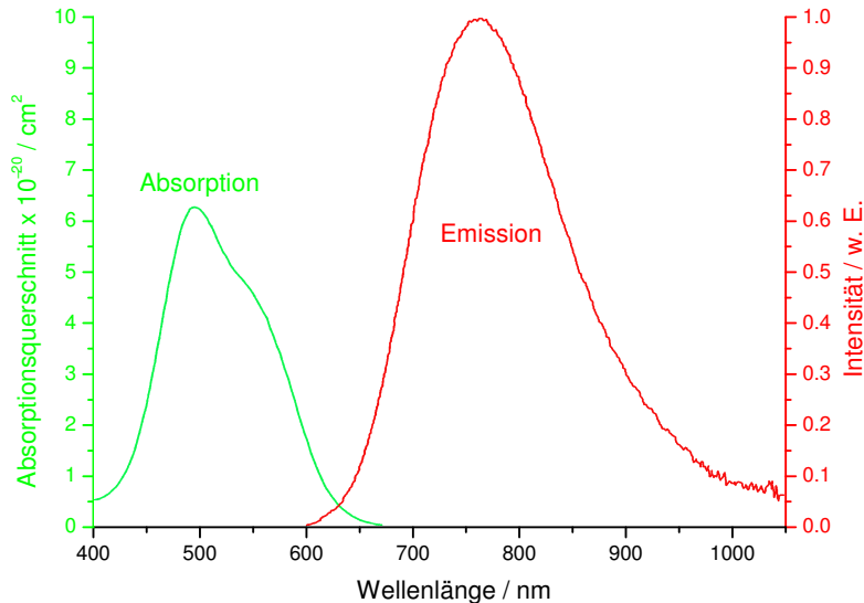
Abbildung 3: Ti:Saphir: Absorptionsbande im Grünen, breitbandige Emission im Roten. Abbildung erzeugt mit Hilfe von Daten aus [1].
