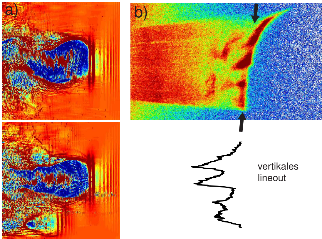
Abbildung 88: a) PIC-Simulationen (ILLUMINATION [212, 213]) zeigen Oszillationen der Elektronen im Rest-Laserfeld innerhalb der Bubble in der Ebene der Polarisationsrichtung (oben), während in der anderen Ebene keine Oszillationen stattfinden. In b) ist ein mit einer Image Plate detektiertes Elektronenspektrum abgebildet, das eine Feinstruktur des Elektronenbunches in der Ebene der Polarisationsrichtung aufweist, die mit der Oszillation zusammenhängen könnte.
