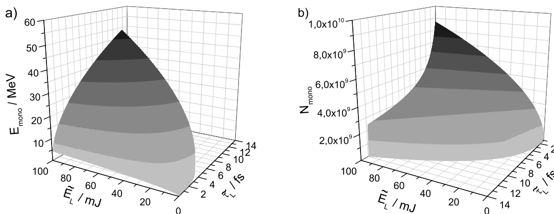
Abbildung 85: Scaling Law-Vorhersage der Energie a) und Elektronenanzahl b) des quasi-monoenergetischen Peaks des Elektronenbunches in Abhängigkeit von den die Bubble treibenden Laserpulsfragmenten.
