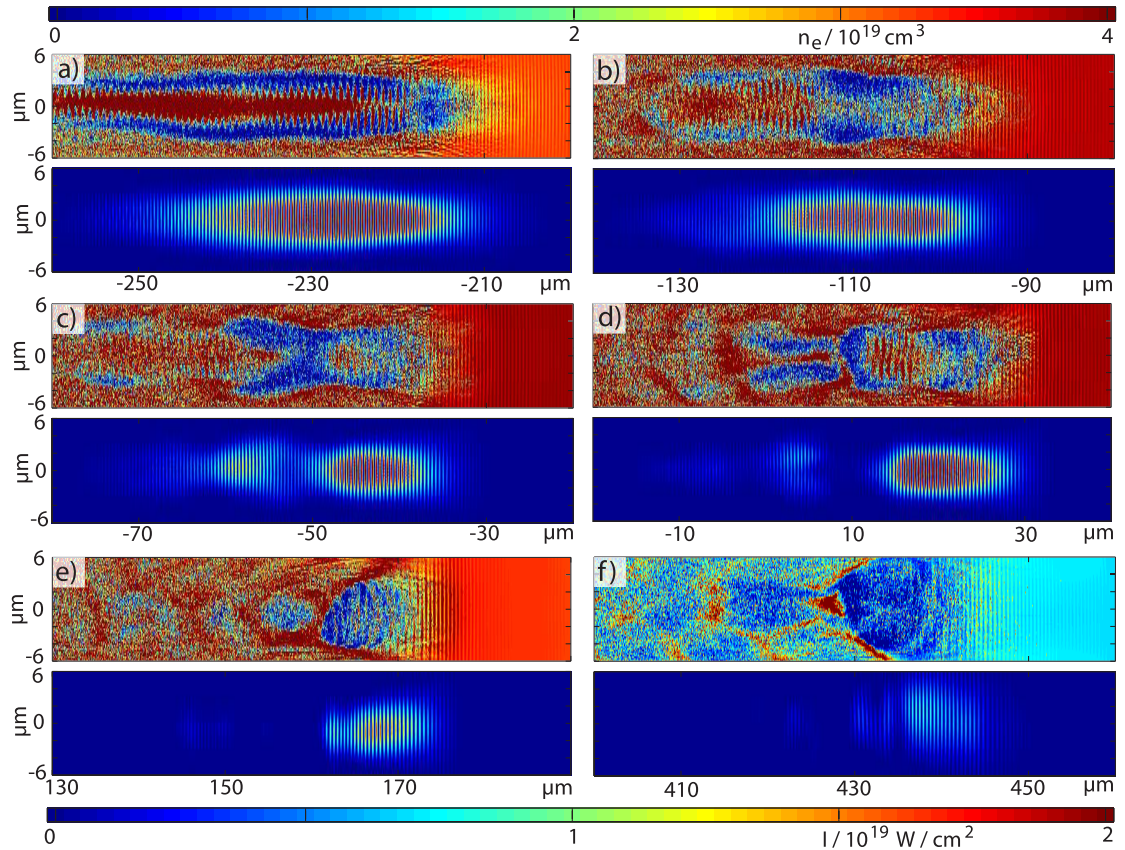
Abbildung 79: Ergebnisse von PIC-Simulationen mit dem ILLUMINATION-Code. Propagation des Laserpulses (jeweils unteres Bild) durch den Gas-Jet mit relativ niedriger Elektronendichte (jeweils oberes Bild) in Höhe von n_e \approx 4 \cdot 10^{19} \text{ cm}^{-3} führt erst spät zur Bildung von Pulsfragmenten und nicht zu effektiver Bubble-Beschleunigung.
