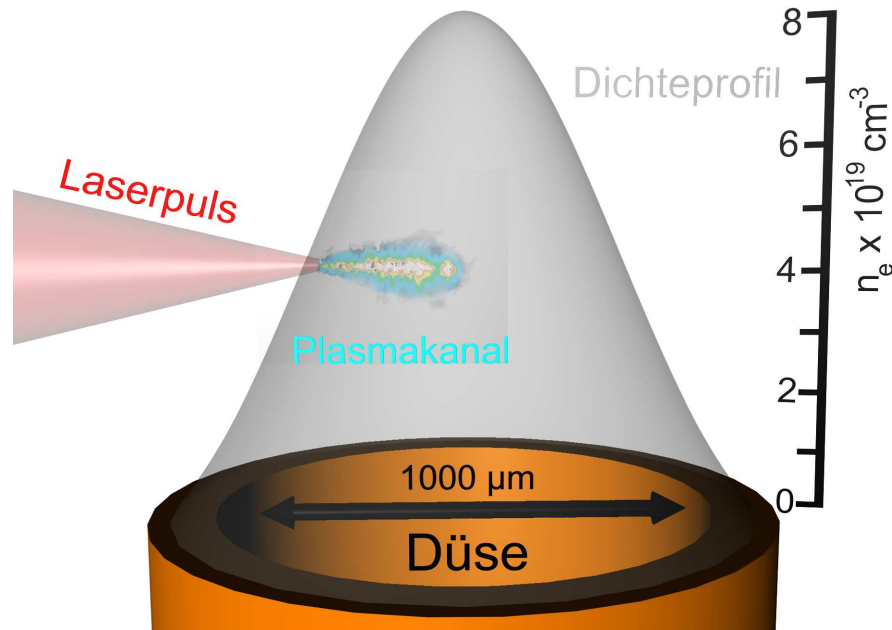
Abbildung 65: Schematische Abbildung zur Bildung eines Plasmakanals im Gas-Jet, der das etwa gaußförmig verlaufende Plasmadichteprofil hat. Der Plasmakanal erstreckt sich in diesem Fall bis etwa zum Dichtemaximum des Gas-Jets. An dieser Stelle hat die Plasmawellenlänge \lambda_p ihr Minimum erreicht und steigt dann wieder an.
