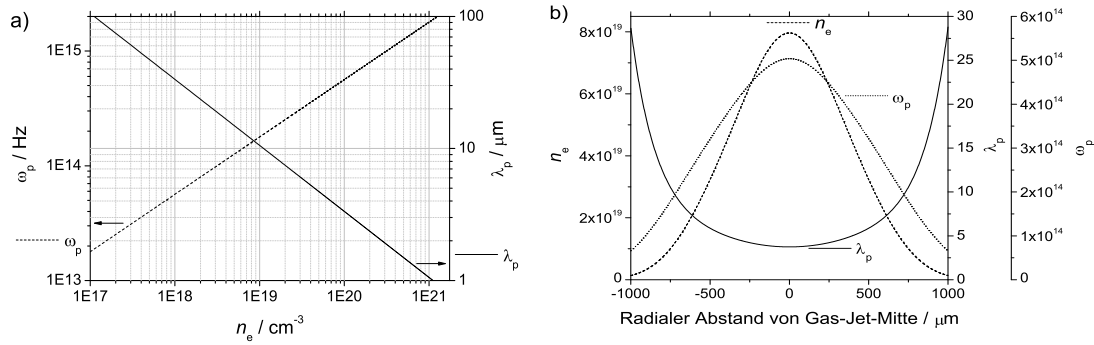
Abbildung 66: a) Überblick über Plasmafrequenz und Plasmawellenlänge bei linear ansteigender Plasmaelektronendichte. b) Ein annähernd gaußförmiges Dichteprofil wie im Experiment mit einem Dichtemaximum bei n_e \approx 8 \cdot 10^{19} \text{cm}^{-3} korrespondiert mit einem deutlich breiteren \lambda_p -Minimum, so dass die Plasmawellenlänge hier über eine große Distanz annähernd konstant bei etwa 4 \mu\text{m} ist.
