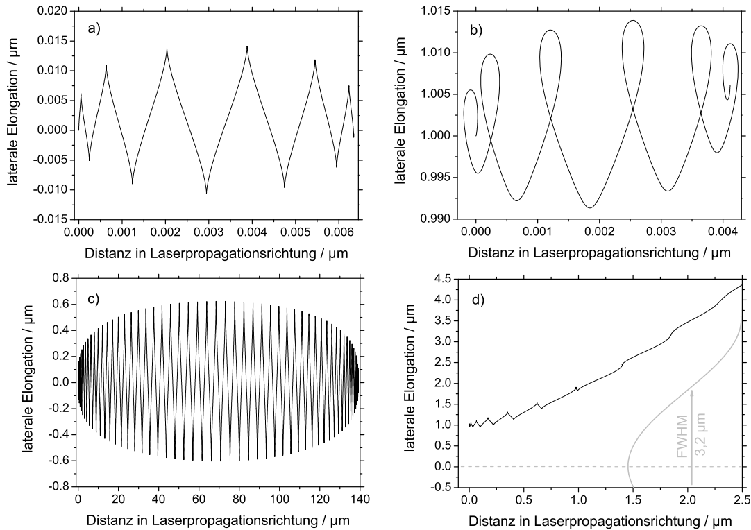
Abbildung 4: Trajektorien von einzelnen, freien Elektronen in Vakuum bei Wechselwirkung mit Laserpulsen. a) Unfokussierter, nicht-relativistischer Laserpuls mit I = 2 \cdot 10^{16} \text{ W/cm}^2 und \tau = 9 \text{ fs} . b) Laserpuls wie in a), aber fokussiert auf einen Durchmesser von 3,5 \mu\text{m} (FWHM). c) Unfokussierter, relativistischer Laserpuls mit I = 5 \cdot 10^{19} \text{ W/cm}^2 und \tau = 80 \text{ fs} . d) Wie c), jedoch fokussiert auf einen Durchmesser von 3,2 \mu\text{m} (FWHM).
