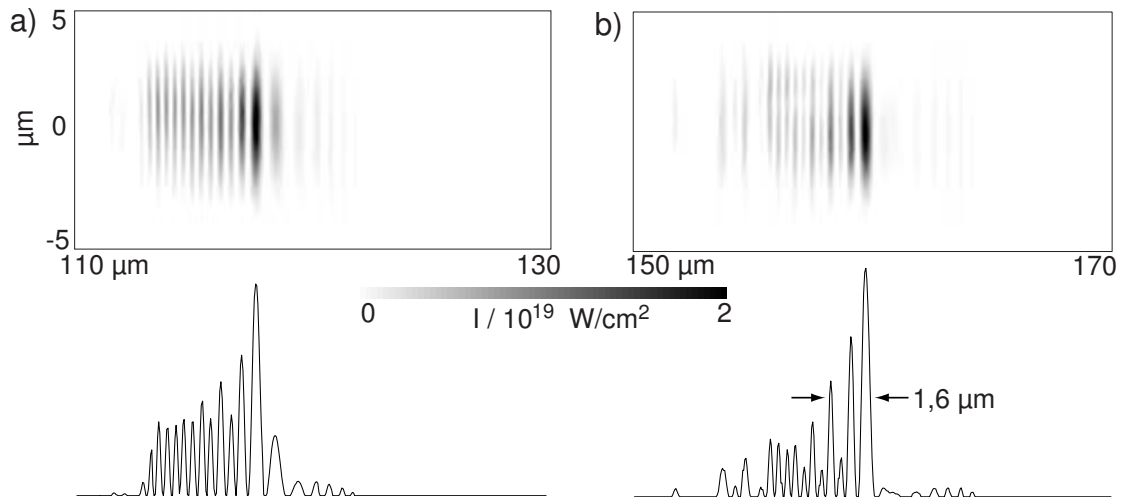
Abbildung 84: a) Laserpulsfragment aus Abbildung 83 h) (oben) und dazugehöriges lineout (unten). b) entsprechend für Abbildung 83 j). Man erkennt deutlich Aufsteilung der Pulsfront, während das Pulsende an Intensität abnimmt.
