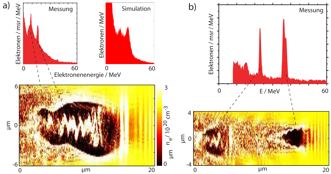
Abbildung 87: Zwei qualitativ unterschiedliche Szenarien zur Bildung von Doppel-Peaks in den Elektronenspektren. a) Bildung aufgrund des Zerfalls eines einzelnen, in einer Bubble beschleunigten Elektronenbunches. Oben links: Gemessenes Spektrum, oben rechts: Spektrum aus einer PIC-Simulation. Dieses Spektrum gehört zum Schnappschuss der Elektronendichte unten im Bild, bei dem sich am hinteren Ende der Bubble ein Teil des Elektronenbunches abspaltet und sich eine wieder aufweitende Plasmastruktur bildet. b) Bildung zweier Bubbles durch selbstmodulierte Laserpulsfragmente. Oben ist ein Messspektrum mit zwei scharfen, deutlich voneinander getrennten und hochenergetischen Peaks abgebildet, unten ein Schnappschuss aus einer PIC-Simulation, in der die Bildung zweier Bubbles angedeutet ist.
