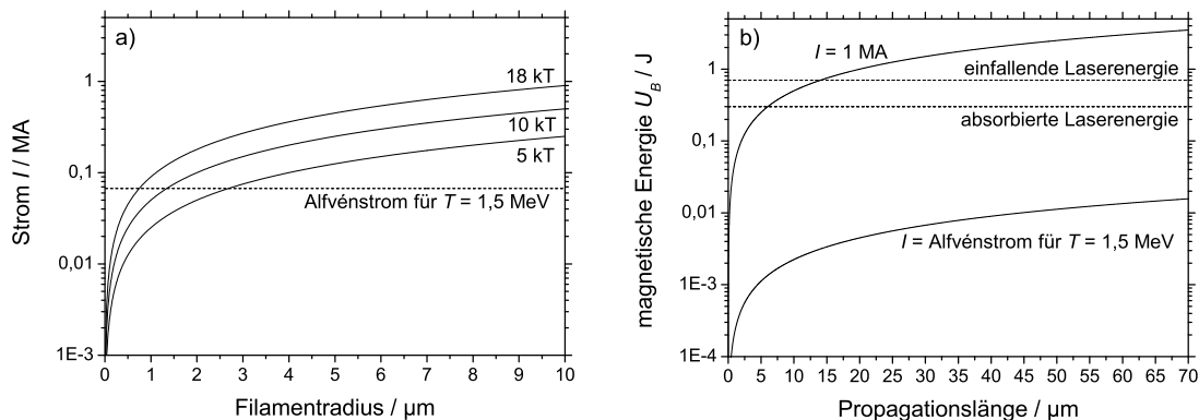
Abbildung 50: a) Strom, der nötig ist, um in einem Filament mit dem Radius r ein Magnetfeld von 18 kT, 10 kT und 5 kT zu erzeugen. Aufgrund des Alfvén-Limits beträgt muss der notwendige Filamentradius deutlich kleiner als der Laserfokus sein. b) Begrenzung der Propagationsdistanz des Nettostroms durch eine Energiebetrachtung.
