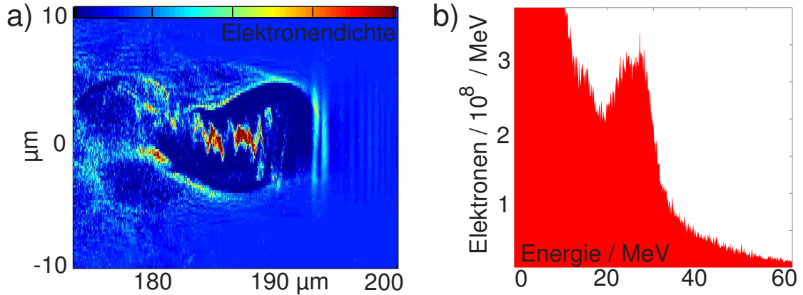
Abbildung 86: PIC-Simulation mit ILLUMINATION für eine den experimentell optimalen Bedingungen entsprechende Plasmadichte: a) Die Dichte der Elektronen ist im Innern der Bubble maximal, und b) diese Elektronen bilden den monoenergetischen Peak im Spektrum bei etwa 30 MeV. Wieder sind alle Elektronen aus der Simulationsbox geplottet, so dass die Zahl der niederenergetischen Elektronen stark ansteigt.
