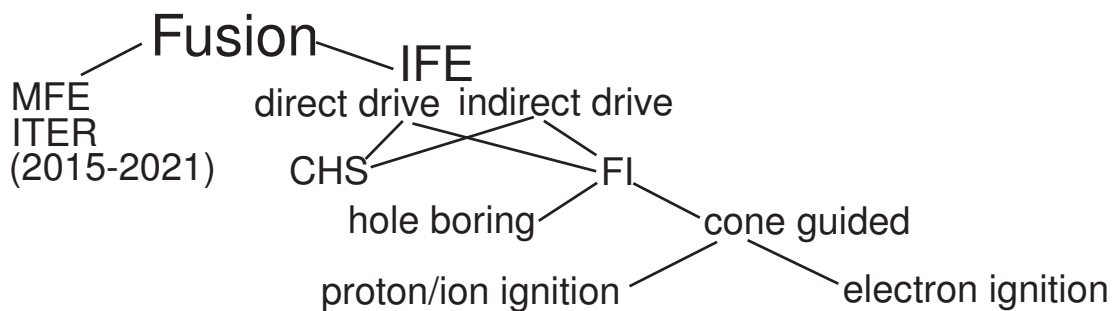
Abbildung 19: Übersicht über diskutierte und angestrebte Fusionsprozesse. Bei der laser-gestützten Inertial Confinement Fusion (IFE) gibt es viele verschiedene Variationen wie Central Hot Spot Ignition (CHS) und Fast Ignition (FI). Die Verwendung von in das Fusionstarget eingesetzten Kegeln (cone-guiding) erlaubt bei der FI je nach Design prinzipiell sowohl die Zündung über Elektronen- als auch über Protonenstrahlen.
