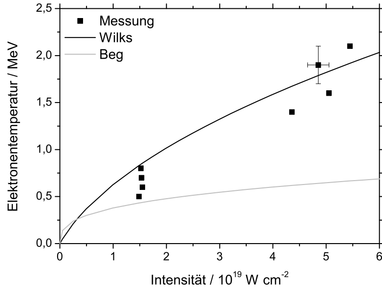
Abbildung 37: Temperaturen der gemessenen Elektronenspektren im Vergleich zu theoretischen Skalierungen in Abhängigkeit von der Intensität. Die Messwerte können durch die Skalierung von [147] (Wilks) sehr gut angenähert werden, während die Skalierung aus [148] (Beg) vor allem für hohe Intensitäten zu kurz greift.
