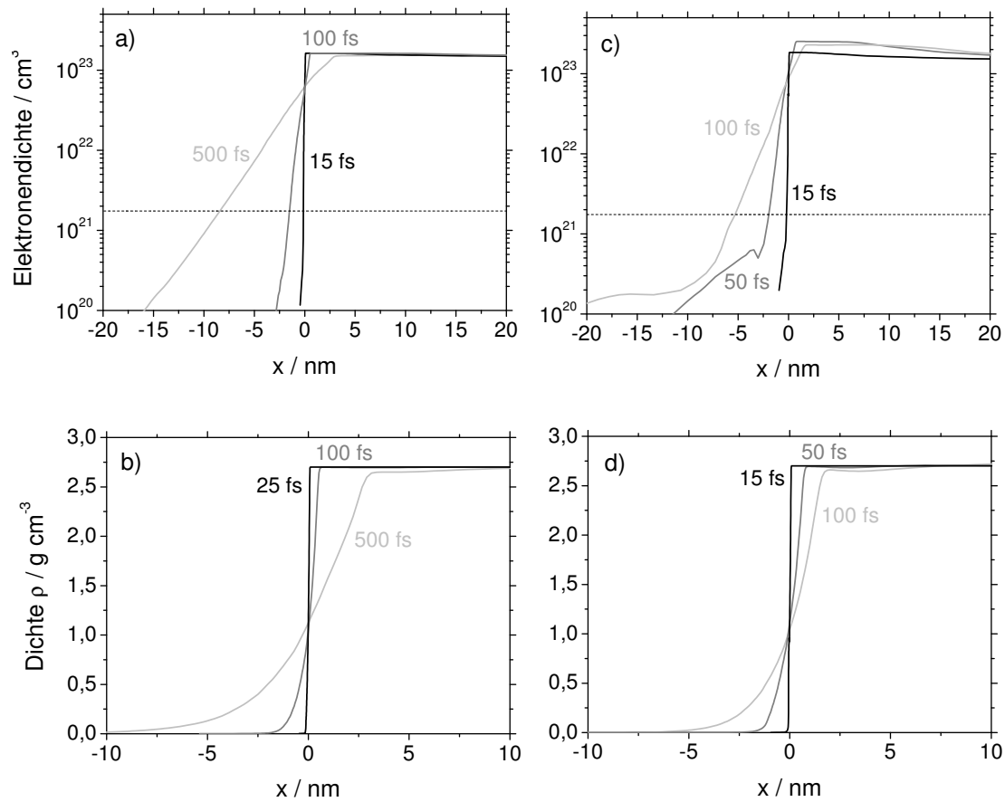
Abbildung 14: Hydrodynamische 1D-Simulationen mit MULTI-FS für einen hypothetischen Laservorpuls (von links kommend, 25 fs Dauer, Targetmaterial: Al). a) und b) zeigen die zeitliche Entwicklung der Elektronen- und Materialdichte für eine Spitzenintensität von 10^{14} W/cm 2 . Analog in c) und d) für 10^{15} W/cm 2 .
