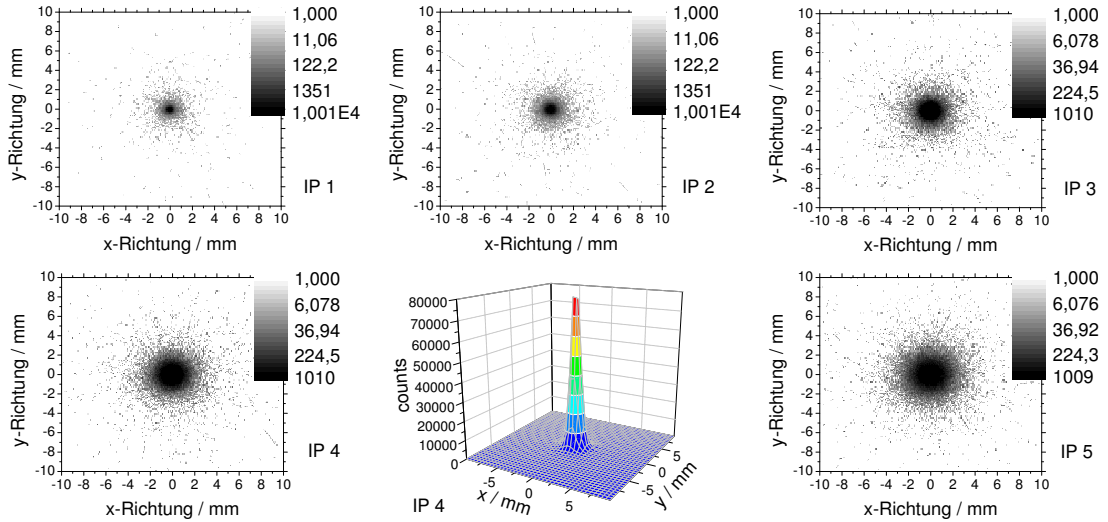
Abbildung 55: Streuung von Elektronen mit einer Energie von E = 20 MeV im IP-Stack.
