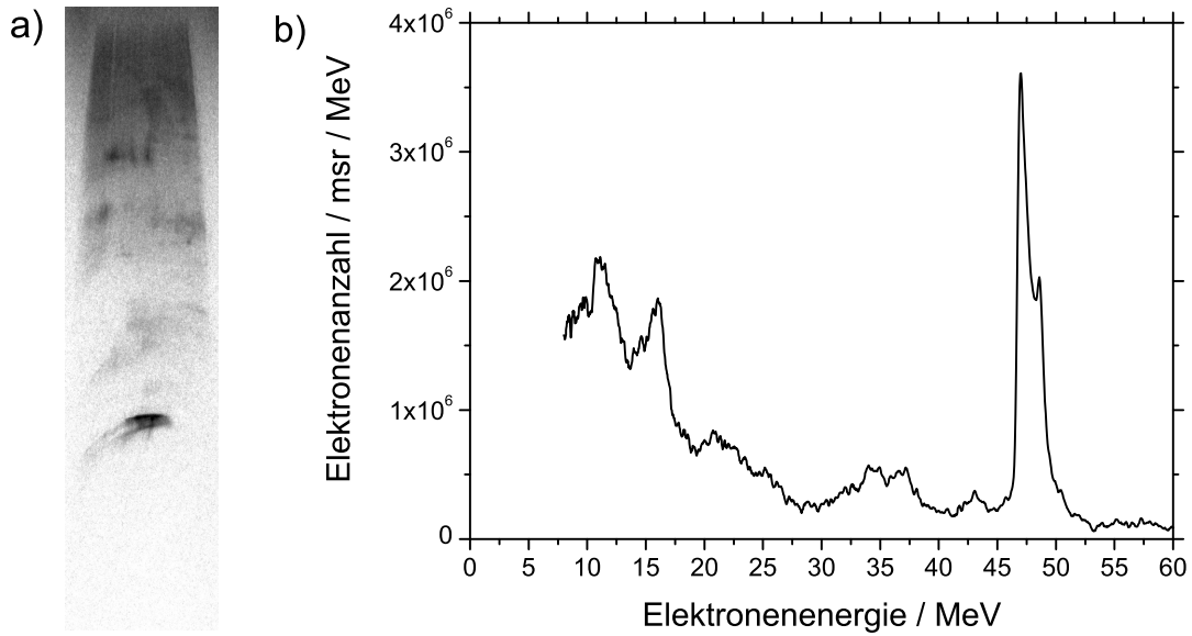
Abbildung 73: a) Rohdaten und b) ausgewertetes Spektrum mit einem monoenergetischen Peak bei einer besonders hohen Energie von ca. 47 MeV (FWHM < 4 MeV).
