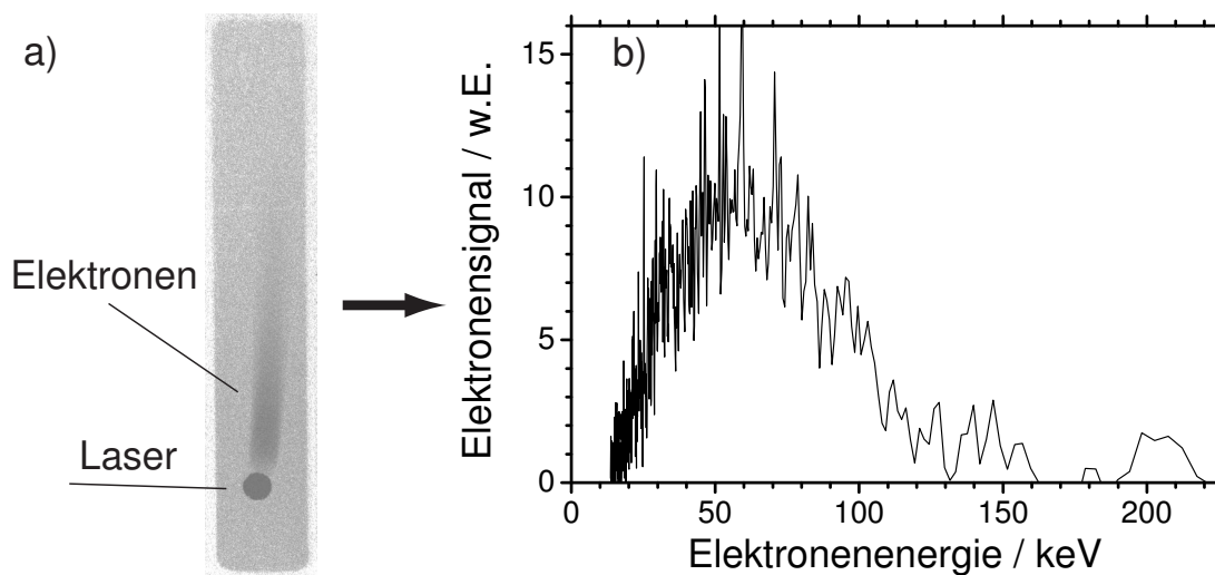
Abbildung 18: Gemessenes Elektronenspektrum für ein Silbertarget. a) Rohsignal auf der IP. b) Ausgewertetes Spektrum (aus [32]).
