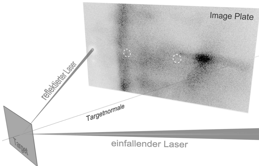
Abbildung 16: Geometrie des Versuchsaufbaus zur Richtungscharakteristik der vom Target emittierten Elektronen. Die Image Plate weist im Bereich zwischen dem reflektierten Laser und der Targetnormalen deutliche Belichtungsmaxima aufgrund gerichteter Elektronen auf.
