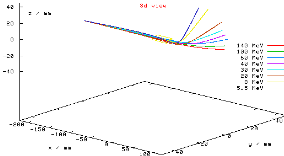
Abbildung 68: Output des selbstgeschriebenen, relativistischen 3D-Trackingprogramms. Die Elektronen verschiedener Energie kommen von rechts und werden durch die vermesenen Randfelder und das zwischen den Magnetplatten existierende B -Feld mit einer Stärke von bis zu 450 mT nach oben hin abgelenkt, wo sich unmittelbar die Detektions-ebene mit der IP anschloss.
