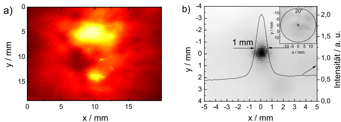
Abbildung 67: Bild des Elektronenstrahls auf dem Beam Viewer bei a) großer Divergenz, die auf eine schlechtere Elektronenausbeute hindeutet, und b) bei sehr geringer Divergenz von \Theta < 10 mrad, was gleichzeitig auf einen hoch- und möglicherweise monoenergetischen Elektronenbunch schließen lässt.
