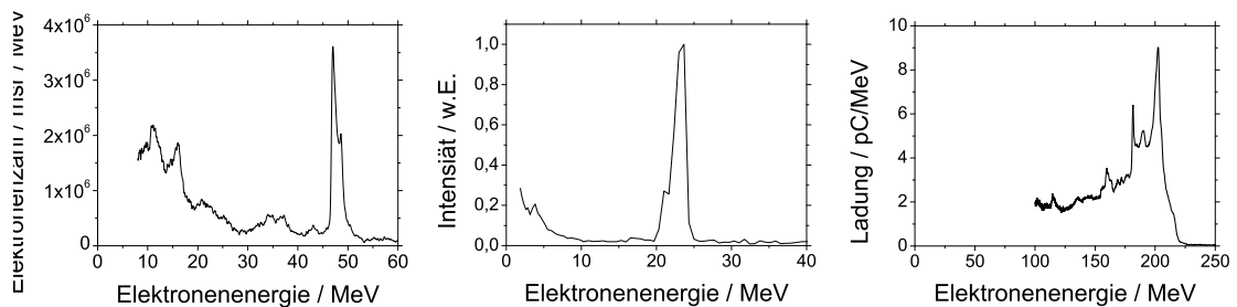
Abbildung 101: Experimentell erhaltene quasi-monoenergetische Elektronenspektren. Links: über das Prinzip der Self-Modulated Laser Wake-Field Acceleration (SMLWFA) mit dem JETI-Laser am IOQ Jena. Mitte: Über das Prinzip der Laser Wake-Field Acceleration (LWFA) mit dem LWS-10-Laser am MPQ Garching. Rechts: Über das Prinzip des aktiven guidings in einer Kapillare mit dem ATLAS-Laser am MPQ Garching. Das Spektrum links wurde im Rahmen dieser Arbeit im Jahre 2004/2005 gemessen. Die damals gewonnenen Erkenntnisse konnten 2007 bei Experimenten am ATLAS- und LWS-10-LASER am MPQ eingebracht werden, an denen der Autor mitbeteiligt war.
