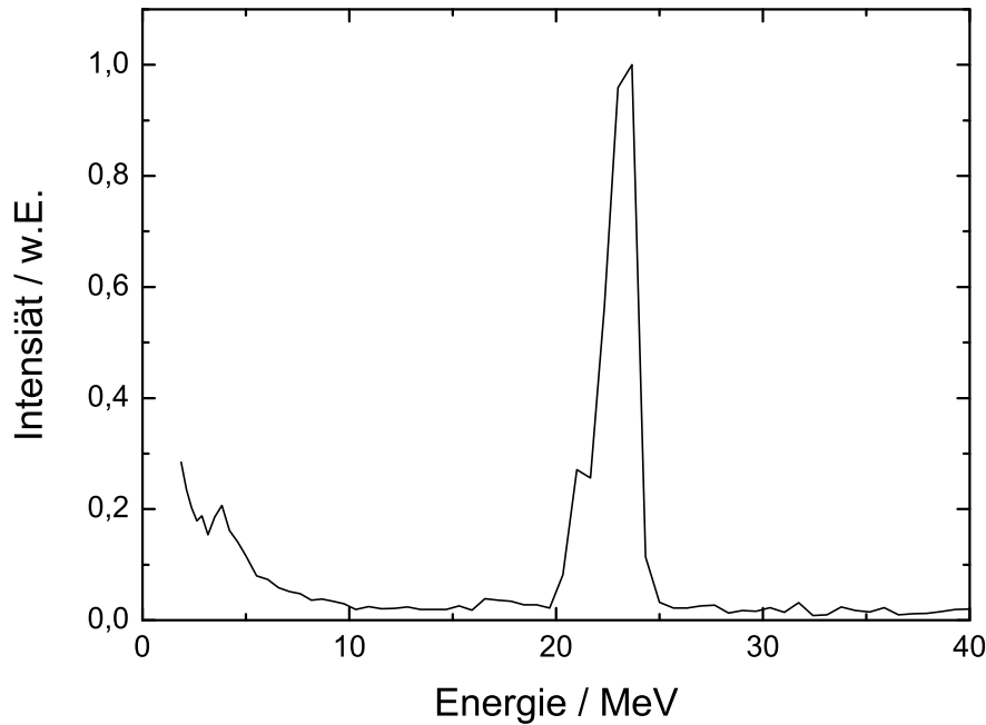
Abbildung 96: Mit dem LWS-10 erzieltes, quasi-monoenergetisches Elektronenspektrum mit einer Energie von etwa 23 MeV mit einer Energiebreite von etwa 2,3 MeV.
