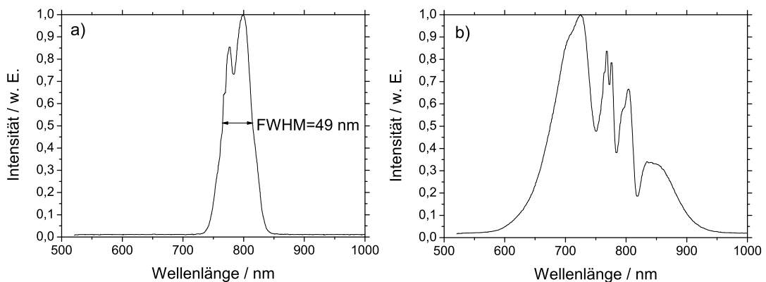
Abbildung 13: Spektrum des Femtopower-Lasersystems vor (a) und nach der Hohlfaser (b).
