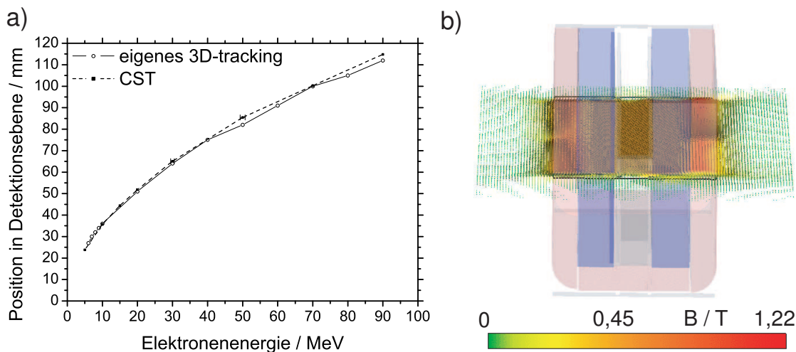
Abbildung 70: a) Direkter Vergleich der mit dem selbstgeschriebenen Tracking-Code und der kommerziellen Software [30] erhaltenen Kalibrierungskurven. Diese stimmen gut überein und bestätigen sich so wechselseitig. b) Ansicht des Spektrometers von schräg hinten und farbkodierter Nachweis dafür, dass das mit der kommerziellen Software errechnete B -Feld auf der Eintrittsachse mit dem gemessenen Wert von 0,45 T übereinstimmt.
