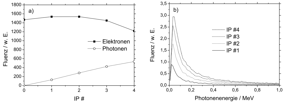
Abbildung 46: Weitere mit dem MULASSIS-Code erhaltene Simulationsergebnisse. a) Vergleich von Elektronen- und dadurch erzeugtem Photonfluss in den Stack-IPs für einen einfallenden Strahl von 5 MeV, b) Energiespektren der dabei generierten Bremsstrahlung.
