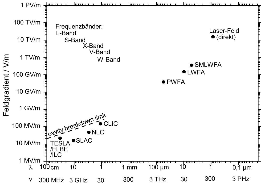
Abbildung 103: Steigerung der elektrischen Beschleunigungsfelder mit steigender Frequenz. Während die Felder herkömmlicher Beschleunigertechnik trotz ausgefeilter Konzepte (zum Beispiel CLIC [295]) im Bereich einiger 10 MV/m liegen müssen (breakdown limit [296]), können durch Laser-Plasma-Konzepte um Größenordnungen höhere Felder ausgenutzt werden. Die höchsten Felder sind die direkten Laserfelder, die möglicherweise durch Interferenzfeld-Beschleunigung an Festkörpern genutzt werden könnten.
