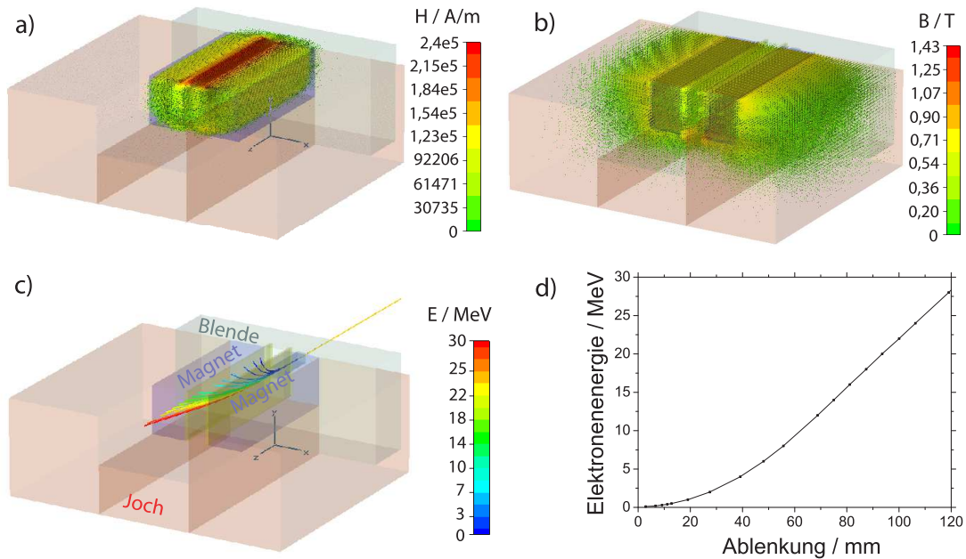
Abbildung 33: Simulationsergebnisse für das Magnetspektrometer für Elektronen bis 30 MeV. a) Von dem Magnetzwilling und dem Joch gebildete H -Feld-Struktur. b) Analog für das B -Feld. Das effektive Feld zwischen den Magneten beträgt etwa 0,23 T. c) Berechnete Trajektorien von Elektronen mit Energien von 0,5 bis 30 MeV beim Durchlaufen dieses Magnetfeldes. d) Ermittelte Energiekalibrationskurve.
