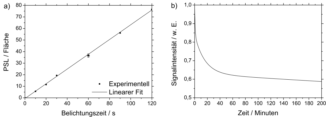
Abbildung 40: Verhalten des Signals auf der Image Plate bei Belichtung. a) Lineare Abhängigkeit des Ausgangssignals der IP vom Eingangssignal. b) Ermitteltes zeitabhängiges fading des Signals auf der IP, hier geplottet nach dem Fit (95).
