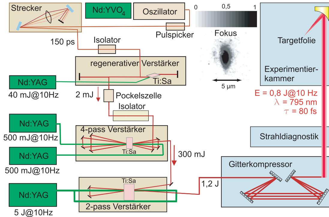
Abbildung 21: Aufbau des Multi-TW-Ti:Sa Lasersystems JETI am IOQ Jena. Durch die Fokussierung des Laserpulses auf einen Fokusspot von etwa 5 \mu\text{m}^2 (FWHM) wurde eine Spitzenintensität von 5 \cdot 10^{19} \text{ W/cm}^2 erreicht.
