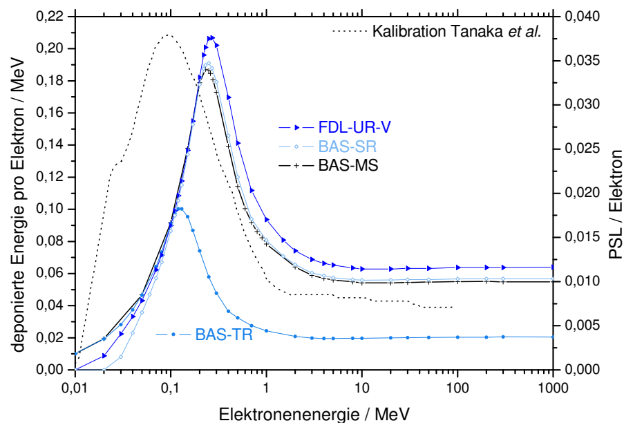
Abbildung 48: Monte Carlo-Berechnung der Elektronenenergie-deposition in sensitiven Schichten verschiedener IPs (durchgezogene Linien, linke y-Achse) und PSL-Kalibrationskurve (gepunktete Linie, rechte y-Achse).
