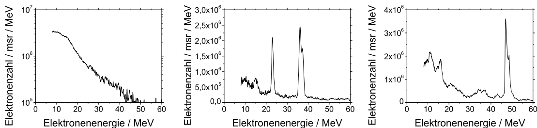
Abbildung 100: Elektronenspektren aus der Self-Modulated Laser Wakefield Acceleration am JETI-Laser. Links: exponentielles Spektrum. Mitte: ausgeprägter Doppel-Peak, der durch zwei hintereinander laufende Bubbles hervorgerufen sein kann. Rechts: quasi-monoenergetisches Elektronenspektrum, bei dem ein einziges, leistungsstarkes Laserpulsfragment den Selbstmodulationsprozess überlebt und eine Bubble treiben kann.
