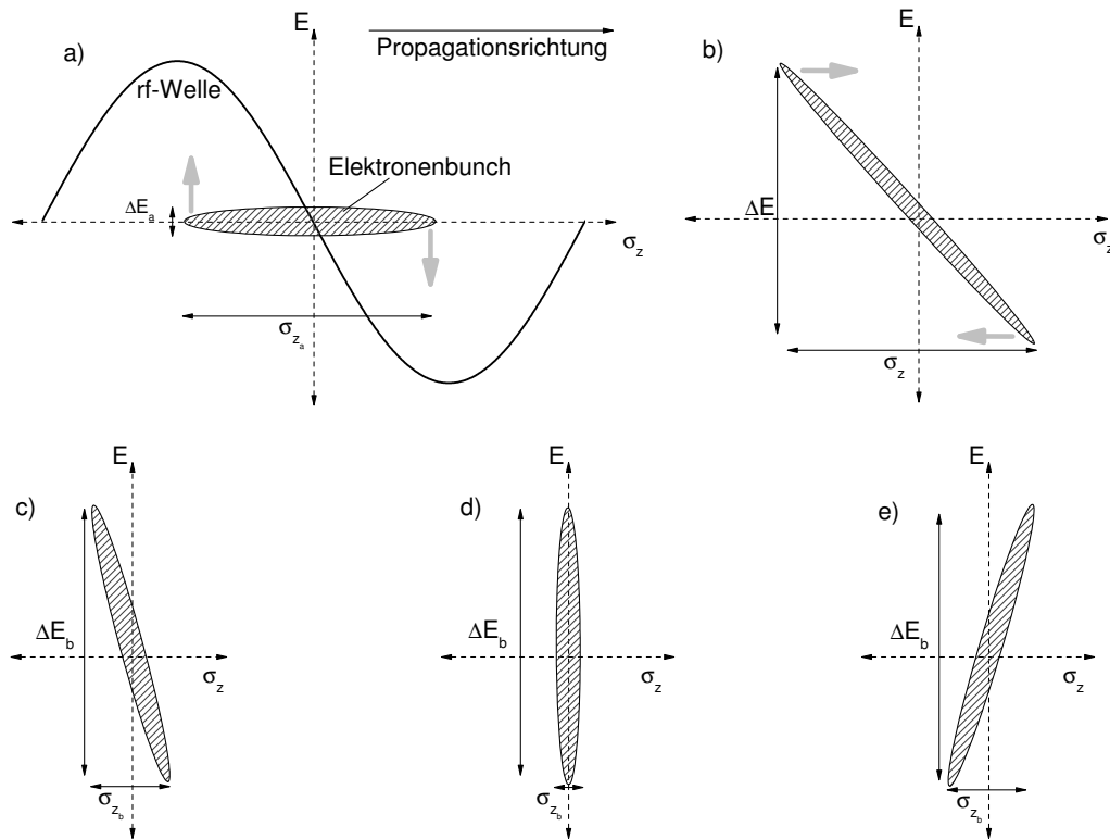
Abbildung 11: Methode zur Pulskompression in konventionellen Beschleunigern. a) Der Elektronenpuls wird durch eine phasenversetzte Beschleunigungswelle energetisch gechipped, die Energiebreite wird erhöht, die Bunchlänge bleibt bestehen. b) Der Puls wird beim Durchlaufen einer Magnetfeld-Schikane aufgrund von Laufzeitunterschieden komprimiert. c) Unterkomprimierter Puls. d) Ideal komprimierter Puls. e) Überkomprimierter Puls.
