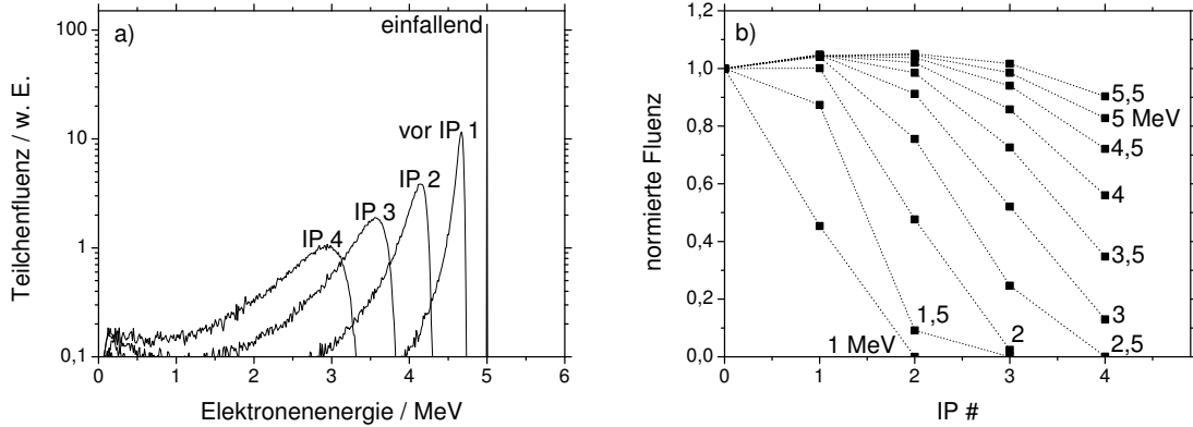
Abbildung 45: Mit MULASSIS erhaltene Simulationsergebnisse für die Änderung des Elektronenflusses beim Durchgang durch den IP-Stack. a) Änderung der Elektronenenergie und des Teilchenflusses mit zunehmender Eindringtiefe in den Stack für einen einfallenden monoenergetischen Elektronenstrahl bei 5 MeV, b) Abnahme des Gesamtflusses mit zunehmender Eindringtiefe für verschiedene Energien.
