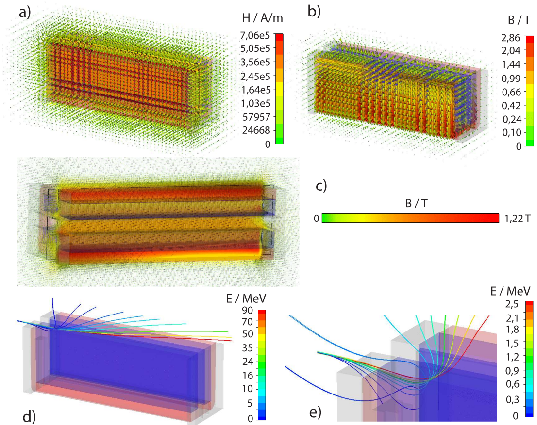
Abbildung 69: Ergebnisse der Simulation des Elektronenspektrometers mit dem CST PARTICLE STUDIO [30]. a), b) und c) zeigt die berechneten Felder, d) und e) die entsprechenden Trajektorien.
