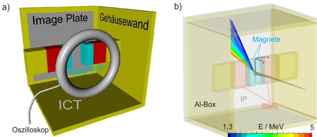
Abbildung 97: Aufbau zur Kreuzkalibrierung von IPs und ICTs bei Laser-Plasma-Experimenten. a) Der einfallende Elektronenstrahl konnte durch eine Blende mit dem Durchmesser 1 cm (nicht eingezeichnet) in das Innere des angedeuteten Gehäuses gelangen, in der er zunächst ein ICT passierte, und dann auf eine an der Rückseite der Box befestigte IP fiel. b) Zuvor konnte der Elektronenstrahl mit Hilfe eines Magnetfeldes leicht aufgespalten werden, so dass sich der Spot auf der IP verbreiterte. Dies dient dem Zweck, eine eventuelle Überbelichtung auf der IP zu verhindern. Das Bild ist ein Ergebnis einer Simulation mit dem CST Particle Studio.
