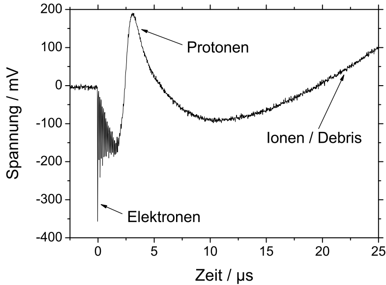
Abbildung 38: Faraday-Cup-Messungen. Typisches Signal vom Faraday-Cup für eine Laserintensität von I_L \approx 2 \cdot 10^{19} \text{ W/cm}^2 .
