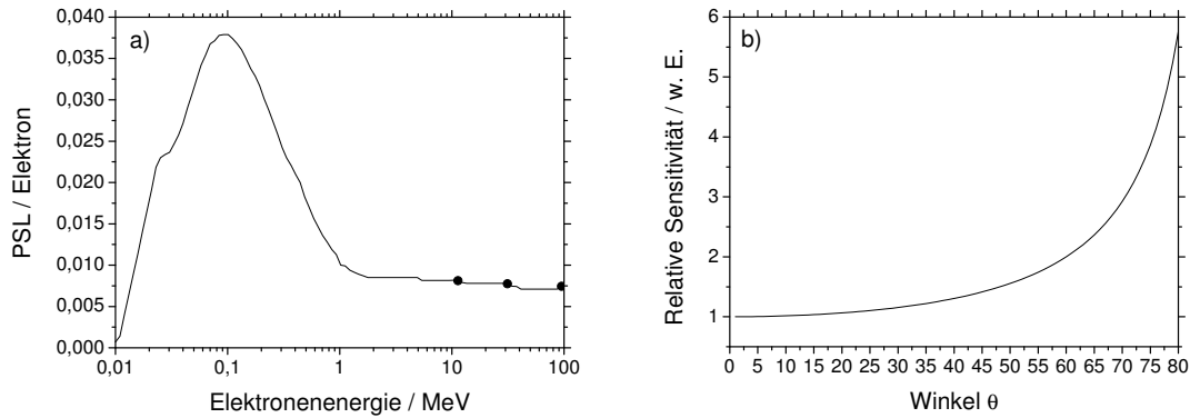
Abbildung 44: Abhängigkeit des Image Plate-Signals von der Energie und dem Einfallswinkel der Elektronen. a) Energie-Kalibrationskurve aus [89]. Die Kalibration beruht auf drei an einem herkömmlichen Beschleuniger erhaltenen Messwerten für Energien zwischen 10 und 100 MeV und früheren Ergebnissen für den darunter liegenden Energiebereich. b) Die Signalintensität steigt mit dem Einfallswinkel \Theta auf die IP wie 1/\Theta an, da die Elektronen dann einen entsprechend längeren Weg durch die sensitive Schicht der IP zurücklegen.
