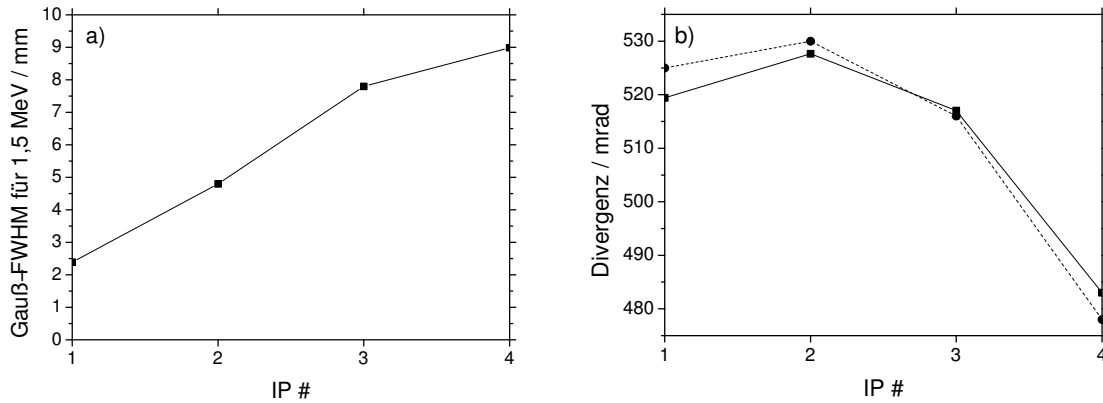
Abbildung 56: a) Aus den Monte-Carlo-Simulationen entnommene FWHM-Gaußbreiten der Elektronenspots in den einzelnen IPs des Stacks aufgrund der Streuung eines Elektronen-Punktstrahls. b) Vergleich der gemessenen und um die natürliche Verbreiterung aufgrund von Streuung entfaltenen Divergenzen.
