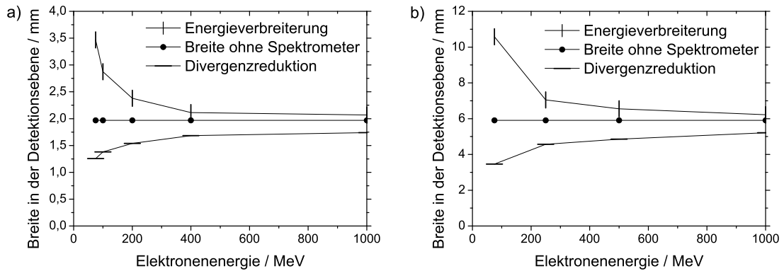
Abbildung 93: Breite des Elektronenbunches nach Durchgang des Elektronenspektrometers in der Detektionsebene im Vergleich zur Breite ohne Spektrometer, nur aufgrund der Strahldivergenz. a) für eine Divergenz von 1 mrad, b) für eine Divergenz von 3 mrad.
