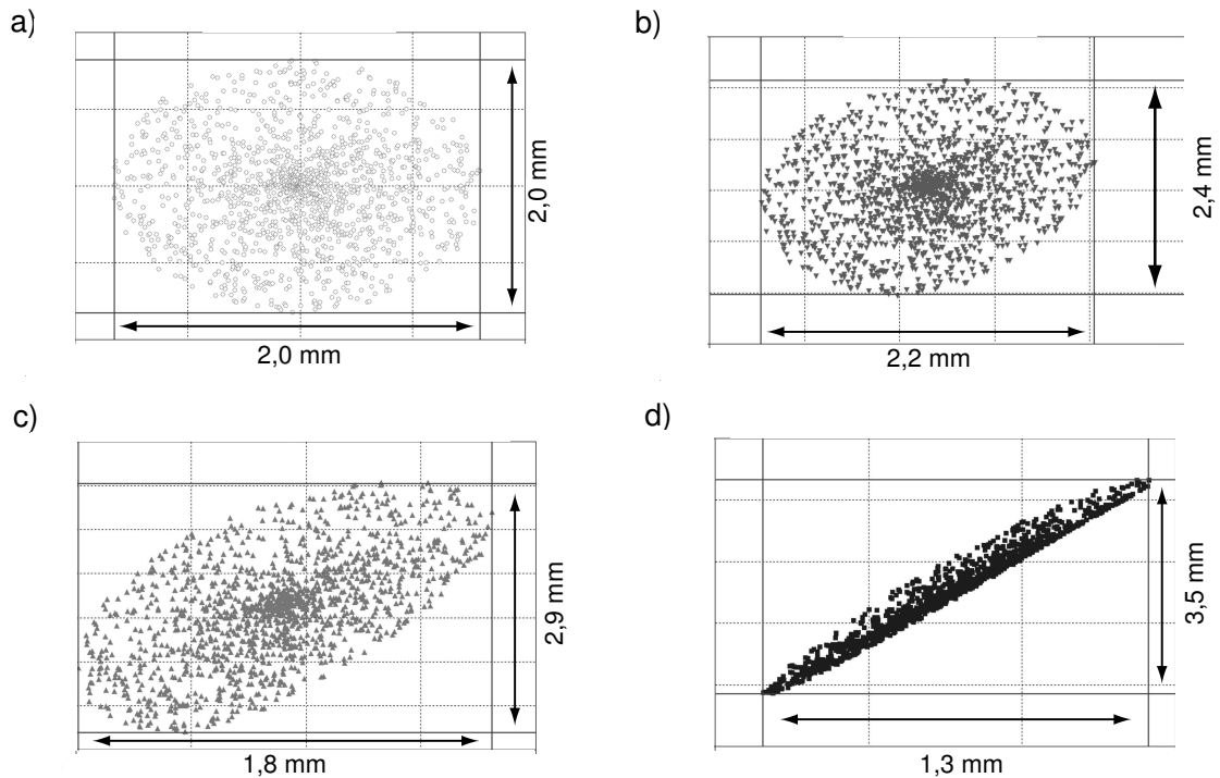
Abbildung 91: Änderung der transversalen Bunchgröße beim Durchgang durch das Spektrometer für einen Bunch der Divergenz 1 mrad und der Energie 75 MeV. a) Unmittelbar vor dem Spektrometereingang, b) in der Mitte des Spektrometers, c) am Spektrometereingang und d) in der Detektionsebene.
