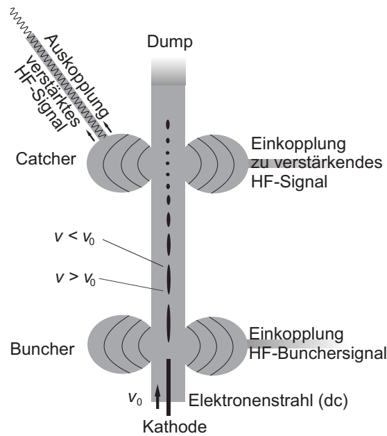
Abbildung 10: Verstärkung einer HF-Welle in einem Klystron zur Einkopplung in den Beschleuniger. Ein Elektronenstrahl wird durch ein Wechselfeld im Buncher geschwindigkeitsmoduliert, so dass einzelne Bunches entstehen, die im Catcher durch eine phasenversetzte HF-Welle abgebremst werden und dadurch einen Teil ihrer Energie an die Schwingung im Catcherresonator abgeben. Die verstärkte Schwingung wird dann durch einen Hohlleiter ausgekoppelt und zum Beschleuniger geleitet.
