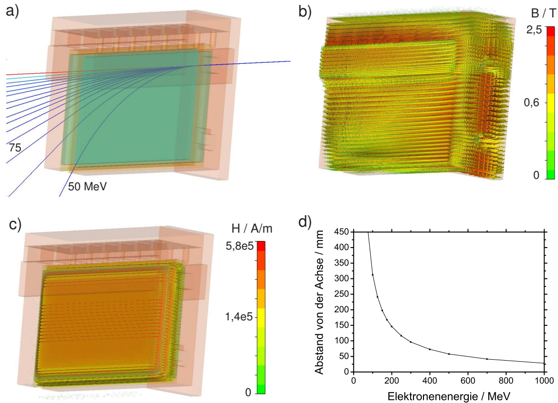
Abbildung 90: Simulationsergebnisse mit CST PARTICLE STUDIO [30] zur Kalibration des bei den Kapillar-Experimenten verwendeten Spektrometers. a) Die Elektronen betreten das Spektrometer von rechts und werden je nach Energie mehr oder weniger stark nach unten abgelenkt. b) und c) zeigen die berechneten Felder, und d) die Kalibrationskurve: Position auf der Detektionsebene vs. Elektronenenergie.
