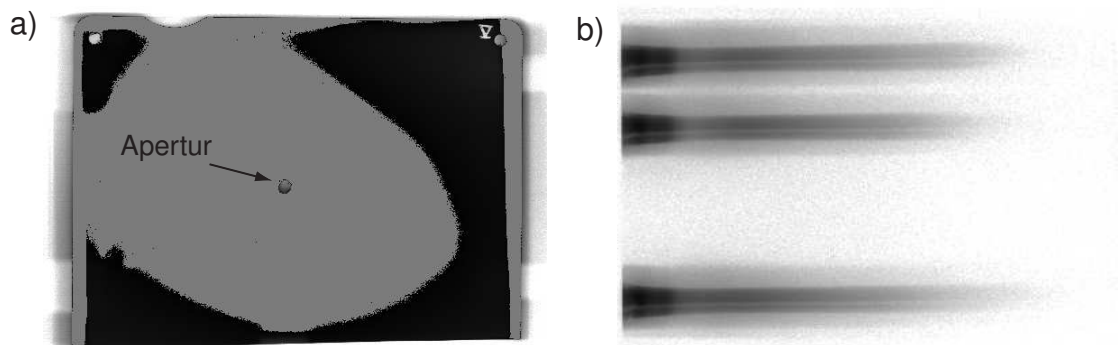
Abbildung 34: Experimentell aufgenommene Image Plate-Bilder. a) Ausgelesene IP vor der Frontabschirmung des Spektrometers mit Eintrittsloch. Die annähernd kreisförmige hellgraue Elektronensignal-Isokontur umschließt das Eintrittsloch zentral. b) Rohdaten der Elektronensignale auf der Detektions-IP hinter der Abschirmung. Die niedrigen Energien befinden sich links auf der IP, die hohen rechts.
