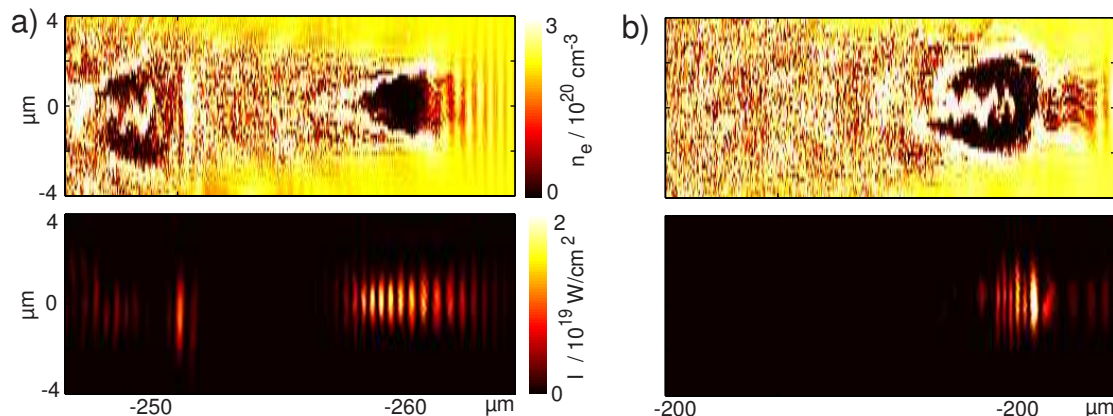
Abbildung 81: PIC-Simulationen mit ILLUMINATION. Details aus Abbildung 80 c) und d) mit anderer Farbskalierung, in der man erkennt, dass a) die beiden vorderen Pulsfragmente jeweils eine Bubble treiben. b) Kurz darauf stirbt die hintere Bubble mit Abklingen dieses Laserpulsfragments ab, während in der vorderen nun Elektronen beschleunigt werden.
