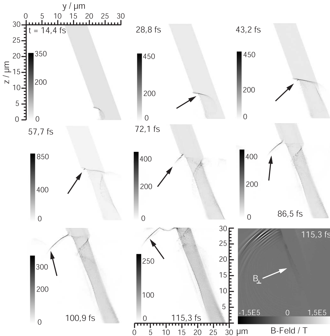
Abbildung 30: Ergebnisse der PIC-Simulation für die Elektronendichte. Die abgebildeten Schnappschüsse zeigen zu denselben Zeiten denselben Ausschnitt wie die in Abbildung 28, nur dass hier statt des E -Feldes die Elektronendichte (in willkürlichen Einheiten) abgebildet ist. Unmittelbar mit dem Aufbau eines Interferenzfeldes bei t = 28,8 fs (siehe dazu Abbildung 28) entsteht ein Elektronenbunch (jeweils mit Pfeilen markiert), der mit dem Interferenzfeld mitwandert und sich verbreitert, während seine Länge (Dauer) sehr kurz bleibt. Hinter dieser Interaktion baut sich an der Targetoberfläche ein starkes quasistatisches, senkrecht magnetisches Feld auf und ist für den letzten zeitlichen Schnappschuss im letzten Bild rechts unten gezeigt.
