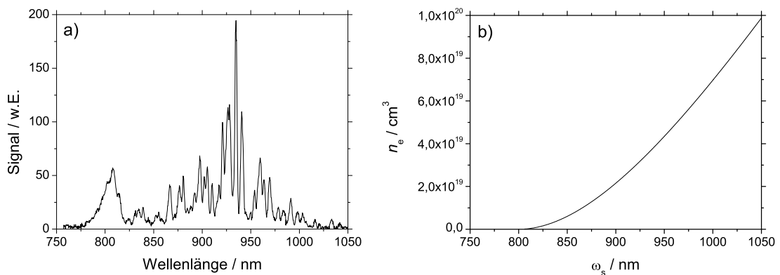
Abbildung 78: Transmittierte Laserspektren. Die Spektren weisen neben dem Peak bei der Zentralwellenlänge des Lasers deutliche Stokes-verschobene Peaks auf, die aufgrund der Selbstmodulation, der Bildung von Laserfragmenten und der variierenden Elektronendichte spektral stark verbreitert sind.
