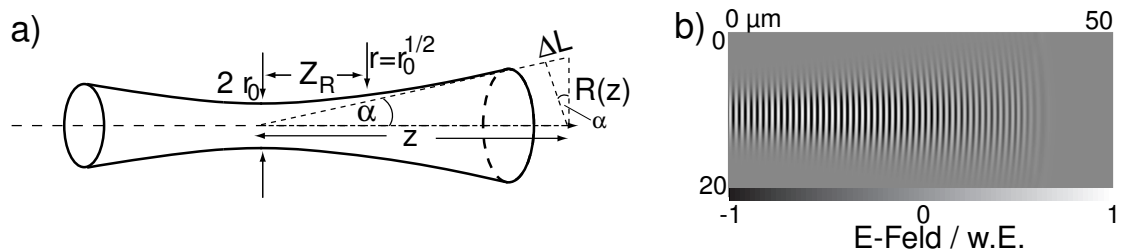
Abbildung 61: a) Schemazeichnung zur Aufweitung eines Gaußschen Strahls durch Beugung. b) PIC-Simulation mit PSC zur Beugung im Vakuum. Es wurde ein 80 fs langer Laserpuls (wie im Experiment), mit einer Breite (FWHM) von 2,5 \mu\text{m} und einer Intensität von I = 2 \cdot 10^{18} \text{ W/cm}^2 von links in die Simulationsbox gesendet. Es ist das E -Feld des Lasers in der Polarisationssebene abgebildet, aus dem man deutlich das Entstehen einer Krümmung der lokalen Wellenfronten durch Beugung erkennt.
