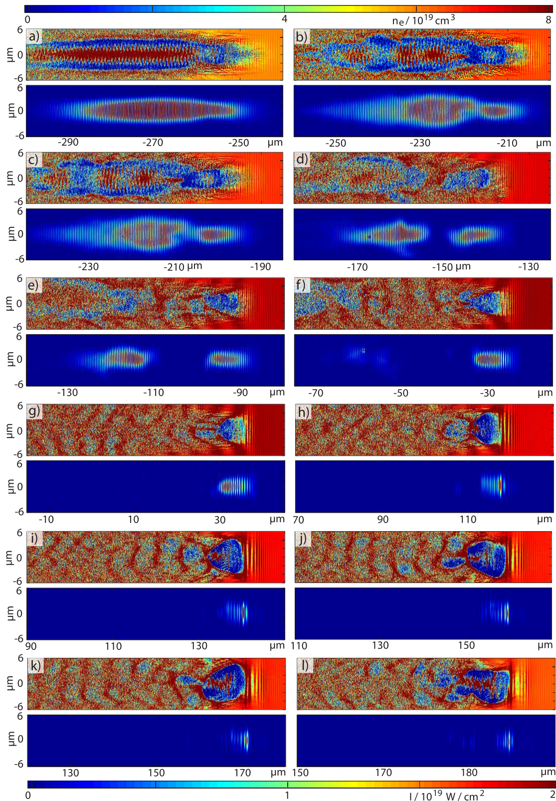
Abbildung 83: PIC-Simulationen mit ILLUMINATION. Bei mittlerer Elektronendichte ähnlich wie im Experiment ( n_e \approx 8 \cdot 10^{19} \text{ cm}^{-3} ) sind Selbstmodulation, Filamentierung und Hosing gemäßigt, aber auch nicht zu schwach, so dass es zur Bildung von Pulsfragmenten und schließlich zur Ausbildung einer relativ stabilen Bubble mit hoher Elektronendichte in ihrem Inneren (jeweils das obere Bild) kommt.
