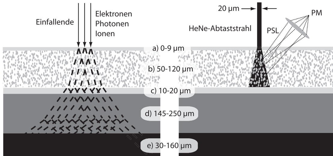
Abbildung 39: Aufbau, Belichtung und Scannen einer Image Plate. Links: Belichtung der IP, etwa durch Elektroneneinfall. Rechts: Auslesen des metastabilen Signals im Scanner, bei dem die He-Ne-Photonen Relaxation der in der sensitiven Schicht angeregten Zustände sowie photostimulierte Lumineszenz (PSL) bewirken, die mit einem Photomultiplier (PM) detektiert wird. Bei beiden Prozessen führt Streuung der Elektronen beziehungsweise der He-Ne-Photonen sowie des PSL-Signals zu einer Signalverbreiterung. Struktur einer IP von oben nach unten: a) Schutzschicht (Mylar), b) sensitive Phosphorschicht, c) Zwischenschicht, d) Grundsicht, e) rückseitige Schicht.
