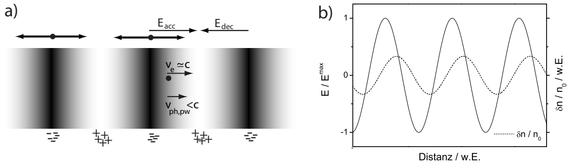
Abbildung 59: a) Schematische Visualisierung des dephasings einer longitudinalen (linearen) Plasmawelle. Während einzelne Elektronen sich mit v_e \approx c nach vorne bewegen können, ist die Phasengeschwindigkeit der Plasmawelle v_{ph,pw} < c , so dass die schnellen Elektronen die beschleunigende Phase der Plasmawelle früher oder später verlassen und keine Energie mehr gewinnen können. b) Dichteüberhöhung (rechte y-Achse) und entsprechende Feldstärke (linke y-Achse) einer solchen linearen Plasmawelle.
