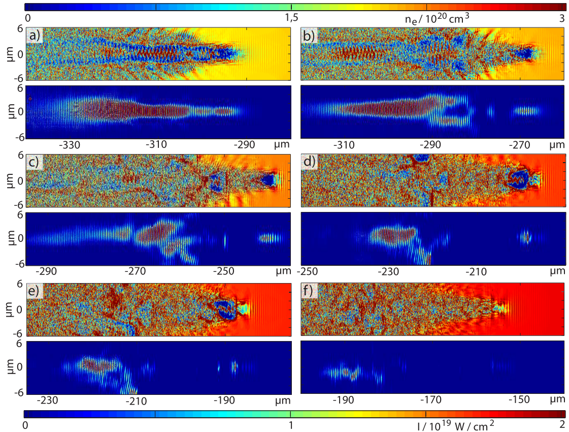
Abbildung 80: PIC-Simulationen mit ILLUMINATION. Bei hoher Elektronendichte ( n_e \approx 3,2 \cdot 10^{20} \text{ cm}^{-3} ) setzt aufgrund der größeren Anwachsrate \Gamma Selbstmodulation des Laserpulses (jeweils unteres Bild) sehr früh ein, führt zu longitudinaler und transversaler Filamentierung und Bildung ein oder sogar zweier Bubbles (siehe c) beziehungsweise vergrößert in Abbildung 81). Es kommt hier noch vor Erreichen des Dichtemaximums zu Laser Depletion.
