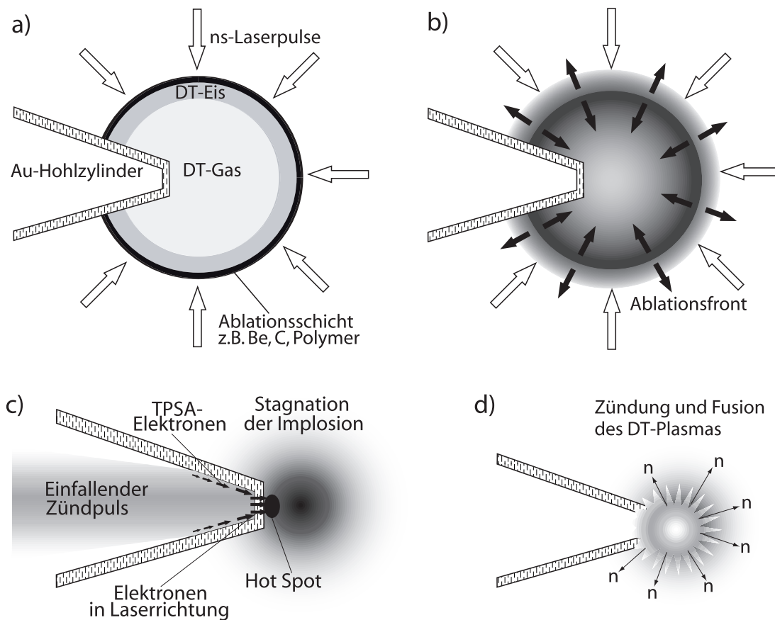
Abbildung 20: Schema der FI nach dem Prinzip des cone-guidings. a) Bestrahlung des Pellets mit mehreren ns-Laserpulsen. b) Raketentypische Kompression des Brennstoffs. c) Der ps-Zündlaserpuls erzeugt Elektronen sowohl an der Oberfläche der Kegelschrägfläche als auch an der Kegelspitze. Diese Elektronen heizen den Hot Spot, der in d) zur Zündung und Fusionsreaktion und Bildung von Neutronen führt.
