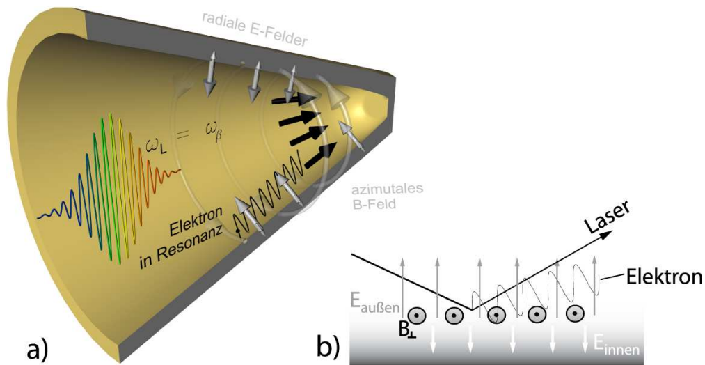
Abbildung 27: a) Erklärung der parallel zur Oberfläche beschleunigten Elektronen über ein der Direct Laser Acceleration verwandtes Prinzip am Beispiel der fusionsrelevanten Hohlkegelgeometrie. Ein relativistisches Elektron schwingt in den elektrischen und magnetischen Feldern (siehe Vergrößerung in b)) resonant mit dem dopplerverschobenen Laserpuls, es kommt dadurch zu Energieübertrag und Vorwärtsbeschleunigung von Elektronen.
