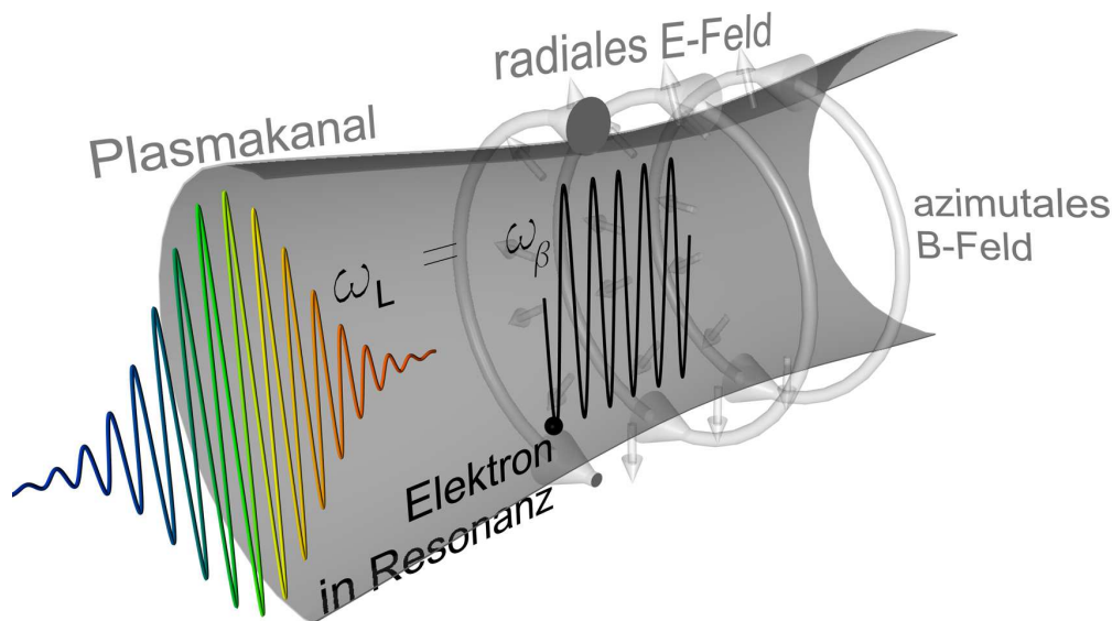
Abbildung 26: Funktionsprinzip der Direct Laser Acceleration (DLA). Das relativistische Elektron schwingt in den selbsterzeugten elektrischen und magnetischen Feldern resonant mit dem Laserpuls, es kommt zu Energieübertrag und Vorwärtsbeschleunigung von Elektronen.
