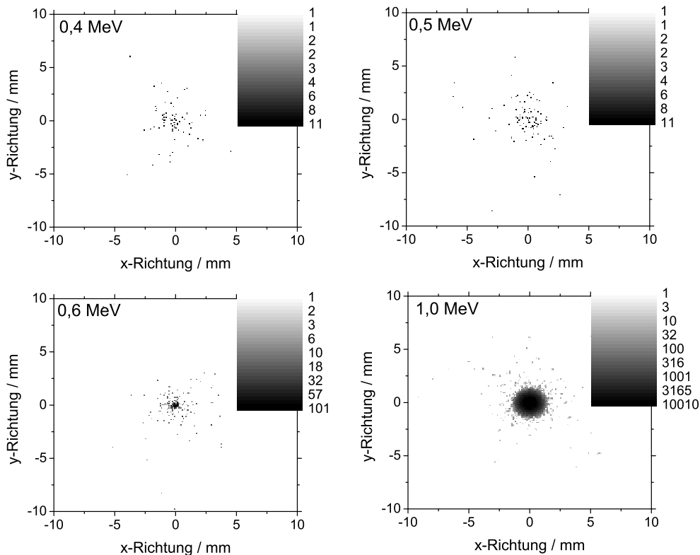
Abbildung 24: Monte Carlo-Simulationen mit GEANT4 zur Streuung von Elektronen verschiedener Energien bei Propagation durch eine Schicht aus 1 mm Aluminium. Erst bei Energien oberhalb von 0,6 MeV kann eine signifikante Anzahl der einfallenden 10^5 Elektronen die Schutzschicht passieren. Gleichzeitig führen Streuprozesse zu einer deutlichen Verbreiterung des einfallenden Punktstrahls. Das Energiespektrum der Elektronen hinter der Aluminiumplatte kann ebenfalls berechnet werden und wird detailliert später behandelt (siehe Abbildung 45).
