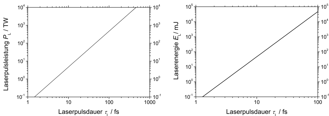
Abbildung 75: Laserleistungs- a) beziehungsweise Energiegrenze b), aber der Bubble-Bildung möglich ist. Plots auf Grundlage von Referenz [230].
