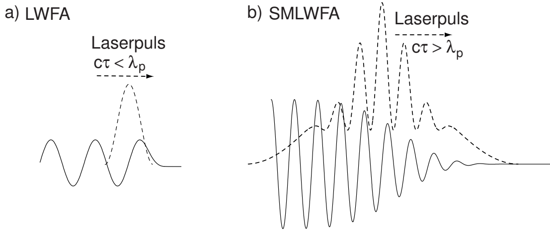
Abbildung 89: Schematischer Vergleich von a) Laser Wakefield Acceleration (LWFA) und b) Self-Modulated Laser Wakefield Acceleration (SMLWFA). Es sind jeweils die Einhüllenden der Laserintensität strichliert gezeigt, während der Dichteverlauf der dadurch angeregten Plasmawelle mit durchgezogenen Linien angedeutet ist. Im Fall der SMLWFA ( c\tau > \lambda_p ) erkennt man, dass im Gegensatz zur LWFA ( c\tau < \lambda_p ) die Einhüllende des Laserpulses mit der Plasmafrequenz moduliert wird.
