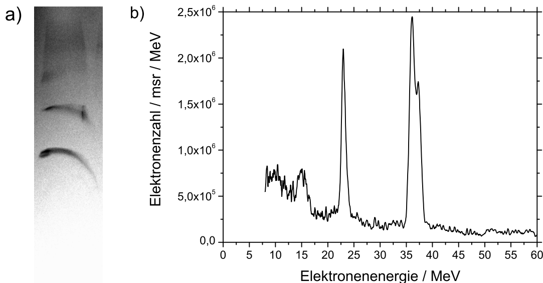
Abbildung 72: a) Rohdaten und b) ausgewertetes Spektrum mit einem sehr scharfen Doppelpeak, hier erhalten unter Verwendung einer subsonischen Düse [228]. Die Energien dieser Peaks liegen bei 23 MeV (FWHM < 1 MeV) sowie bei 36 MeV (FWHM < 2 MeV).
