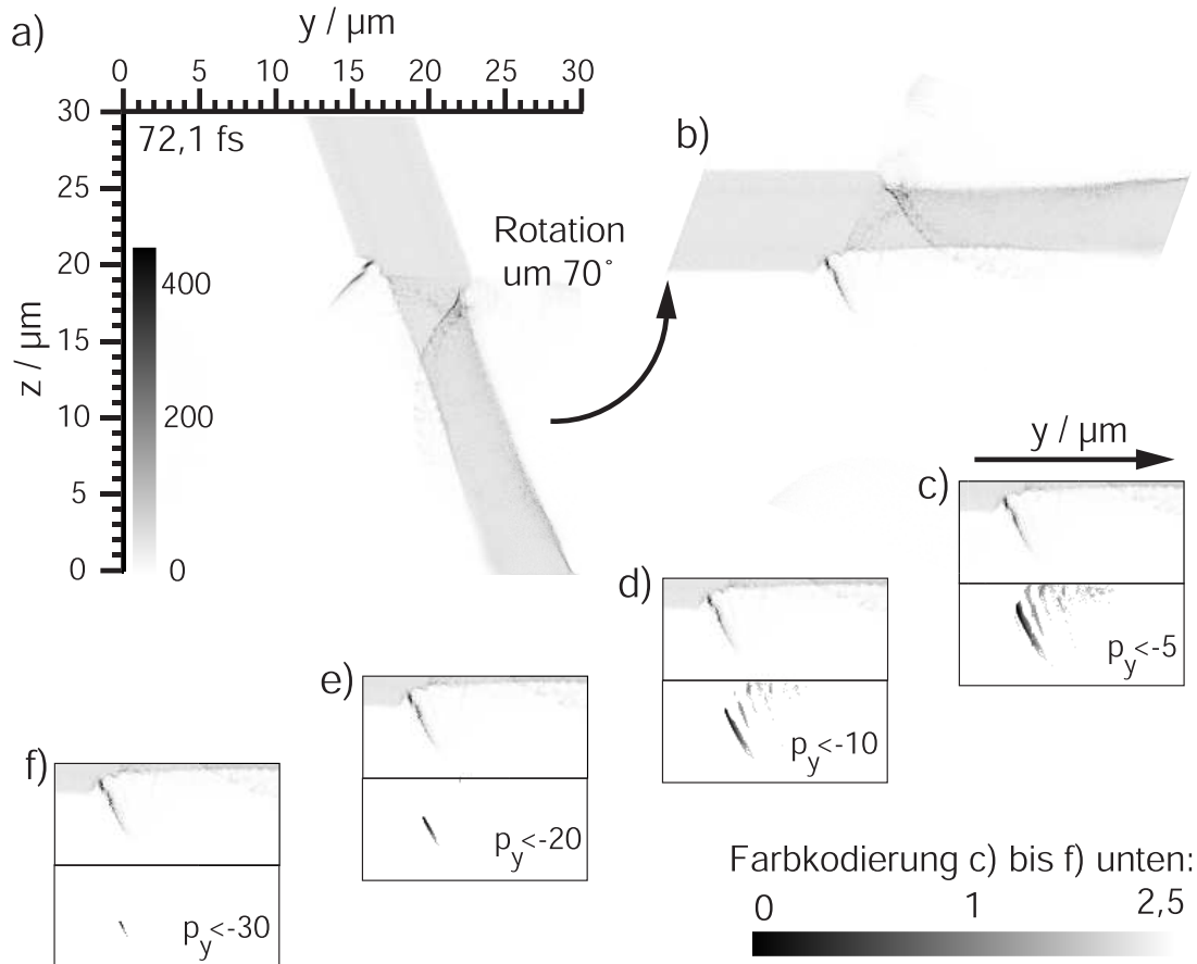
Abbildung 32: PIC-Simulation (PSC): a) Schnappschuss der Elektronendichte bei t = 72,1 fs, b) Elektronendichte gedreht um 70^\circ , c) bis f) die zentrale Wechselwirkungszone mit Plots der Elektronendichte (jeweils oben) und (mit einer anderen (logarithmischen) Farbkodierung) ausschließlich diejenigen Elektronen, die einen bestimmten Impuls parallel zum Target überschreiten. Es ist erkennbar, dass es sich um einen ganzen Pulszug ultrakurzer Elektronenbunches (c) handelt, von denen der zuerst beschleunigte Teil am weitesten außen sitzt und am meisten Beschleunigungsenergie aufgenommen hat.
