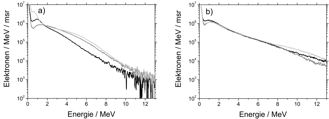
Abbildung 35: Gemessene Elektronenspektren in Vorwärtsrichtung bei a) einer Intensität etwas unterhalb von I_L \approx 5 \cdot 10^{19} \text{ W/cm}^2 und einer 2 \mu\text{m} dicken Titanfolie als Target, b) einer Intensität etwas oberhalb von I_L \approx 5 \cdot 10^{19} \text{ W/cm}^2 und einer 5 \mu\text{m} dicken Titanfolie.
