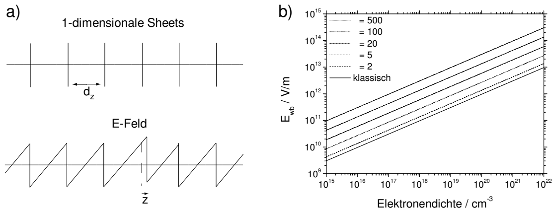
Abbildung 58: Historische Modellierung des Wellenbrechens nach Dawson und Wave-Breaking-Limits nach Akhiezer und Polovin. a) Eindimensionales Plasma-Sheet-Modell nach [169]. Oben: Die einzelnen, negativ geladenen Sheets befinden sich im Gleichgewichtszustand in äquidistanten Abständen \delta_z über einem fixierten, positiv geladenen Ionenhintergrund. Unten: Das sich daraus ergebende sägezahnförmige E-Feld ändert sich bei Variation der Position eines Sheets, wobei die wechselseitige, gekoppelte Änderung des Feldes vom Computer berechnet werden kann. b) Die Plasmawelle kann nur eine bestimmte Feldstärke aushalten, ohne zu brechen. Der Graph zeigt entsprechende (relativistische) Wave-Breaking-Limits nach [170].
