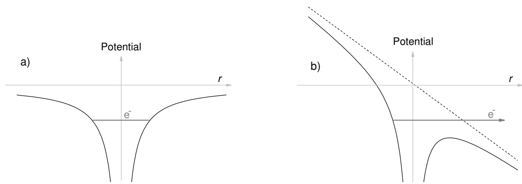
Abbildung 6: Verzerren des Bindungspotentials eines Elektrons in einem Atom durch einen intensiven Laserpuls. In a) ist das Bindungspotential ungestört, in b) ist es durch das E -Feld des Laserpulses so weit verformt, dass das vorher gebundene Elektron den Atomverbund verlassen kann (ABI).
