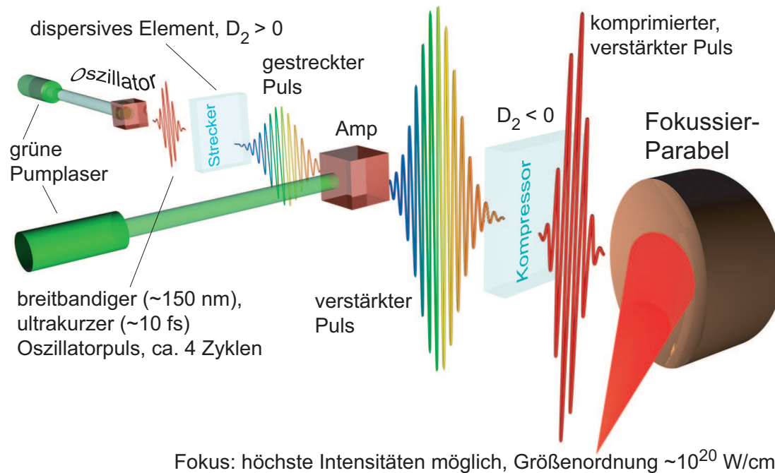
Abbildung 2: Schematische Zusammenfassung der Prozesse, die zur Erzeugung der gewaltigen elektromagnetischen Felder führen, die in der Laser-Plasma-Beschleunigung ausgenutzt werden.
