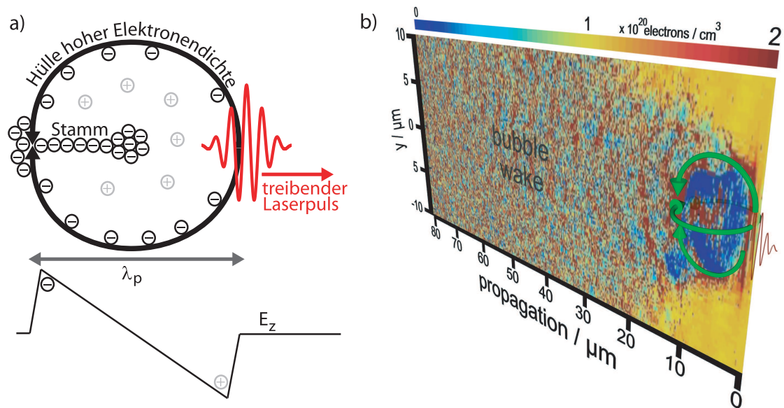
Abbildung 63: a) Schematische Darstellung der Bubble-Bildung. Elektronen werden vom treibenden Laserpuls zunächst von der Achse vertrieben, bilden eine elektronenfreie sphärische Kavität, in der ein longitudinales E -Feld E_z mit abgebildetem Verlauf existiert. b) Visualisierung einer geformten Bubble auf Grundlage einer 3D-PIC-Simulation (ILLUMINATION-Code [212, 213]).
