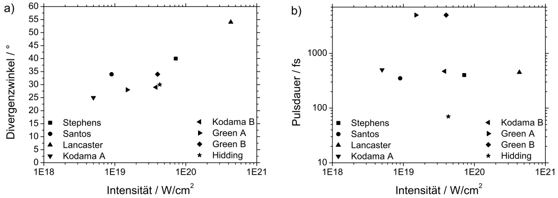
Abbildung 57: Divergenz der für in Vorwärtsrichtung beschleunigte Elektronen bei Laser-Festkörper-Experimenten für verschiedene Laserparameter. a) Intensitätsabhängigkeit der Divergenz der Elektronenstrahlen für relativistische Laserintensitäten. b) verdeutlicht, dass das Scaling auf sub-100-fs erweitert werden kann. Quellen: Stephens [160], Santos [161], Lancaster [162], Kodama A [76], Kodama B [92], Green A [159], Green B [159], Hidding.
