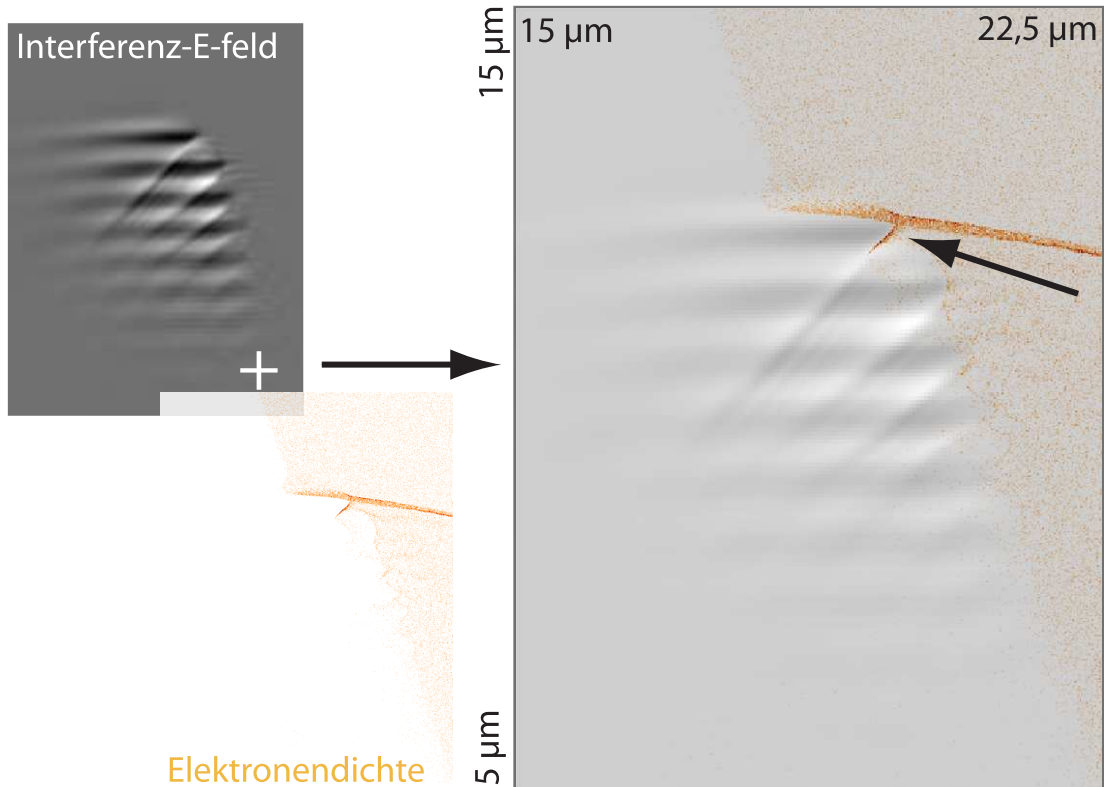
Abbildung 31: PIC-Simulation (PSC): Schnappschuss der Beschleunigung eines Elektronenbunches im Interferenzfeld eines an der Festkörperoberfläche reflektierten Laserpulses. Die Einzelbilder (links) für das E -Feld und für die Elektronendichte bei t = 43,2 fs sind rechts in der Abbildung kongruent übereinander gelegt worden, so dass erkennbar ist, dass sich der Elektronenbunch genau in einer Phase des E -Feldes befindet, in der das E -Feld gerade ansteigt. Der Elektronenbunch muss daher hier entsprechende beschleunigende Felder der Größenordnung 10 TV/m erfahren (siehe Abbildung 29).
