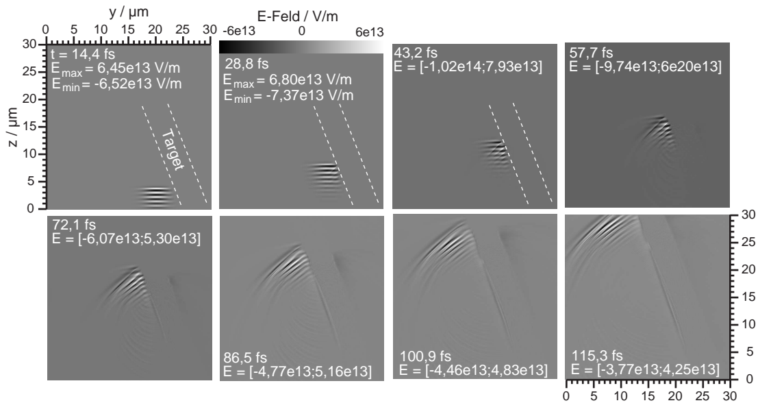
Abbildung 28: PIC-Simulation mit dem PLASMA SIMULATION CODE PSC [112]. Es sind Schnappschüsse des E -Felds des von unten kommenden Laserpulses im Abstand von 14,4 fs gezeigt. Die Reflektion an der Targetoberfläche führt zur Ausbildung eines Interferenzfeldes und zu Feldüberhöhung, besonders deutlich bei t = 43,2 fs in Bild 3.
