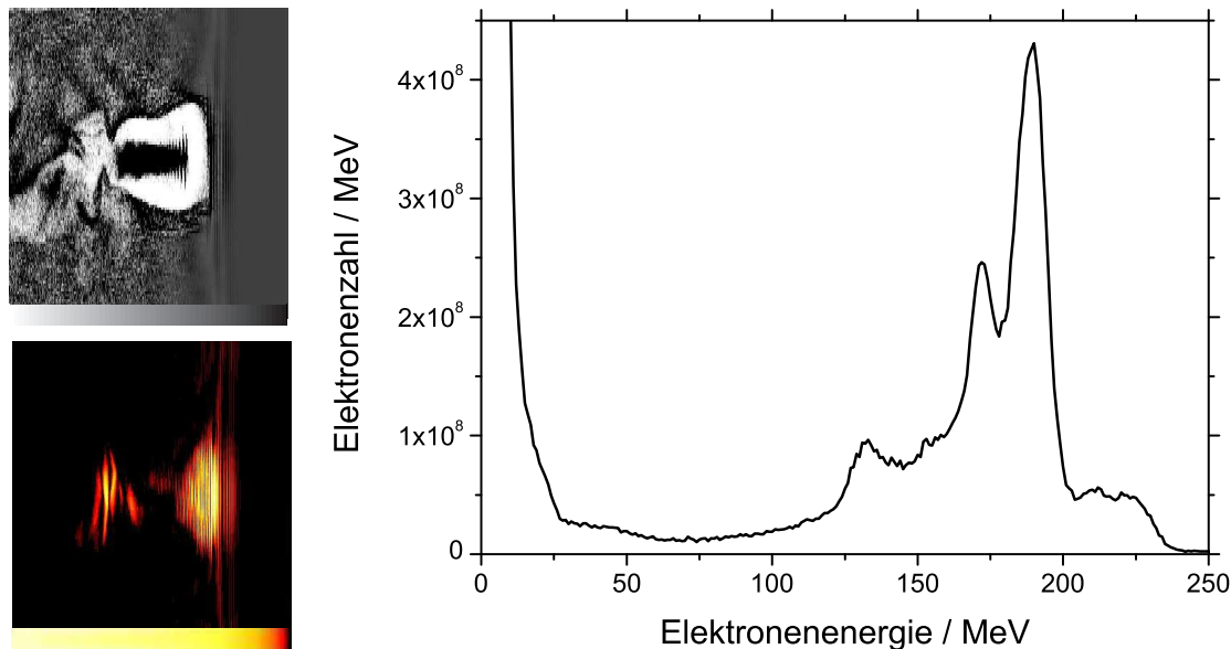
Abbildung 104: Erste Simulationsergebnisse mit dem VLPL-Code von A. Pukhov [261] für Bubble Acceleration mit dem neuen Düsseldorfer 100 TW-Lasersystem mit einer Pulsdauer von unter 25 fs. Links oben: Momentaufnahme einer ausgeprägten Bubble mit hoher Elektronendichte im Innern (in der Polarisationssebene). Links unten: Laserintensität in der Polarisationssebene zu derselben Zeit. Rechts: Entsprechendes Elektronenspektrum mit einem starken Peak bei etwa 200 MeV. Es sind alle Elektronen aus der Simulationsbox berücksichtigt worden.
