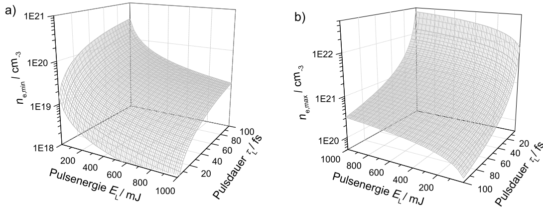
Abbildung 74: Minimale a) beziehungsweise maximale b) Dichte in Abhängigkeit von Pulsenergie und Pulsdauer, bei der Bubble-Bildung möglich ist.
