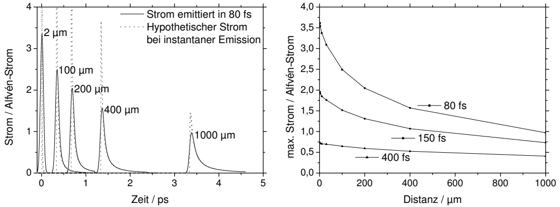
Abbildung 51: a) Auf das (herkömmliche) Alfvén-Limit normierter Strom für die gemessene Ladung und Temperatur in Abhängigkeit von der Distanz vom Target für instantane Emission (gestrichelte Linie) und Emission innerhalb von 80 fs (durchgezogene Linie). b) Strom im Falle größerer effektiver Emissionsdauern vs. Distanz vom Target.
