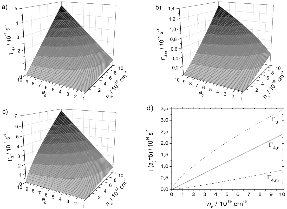
Abbildung 76: a)-c) Anwachsrate \gamma_0 der RFS-Instabilität nach Gleichungen 155 bis 157 für verschiedene n_e und a_0 sowie für die im Experiment verwendete Vakuumintensität a_0 = 5 in d).
