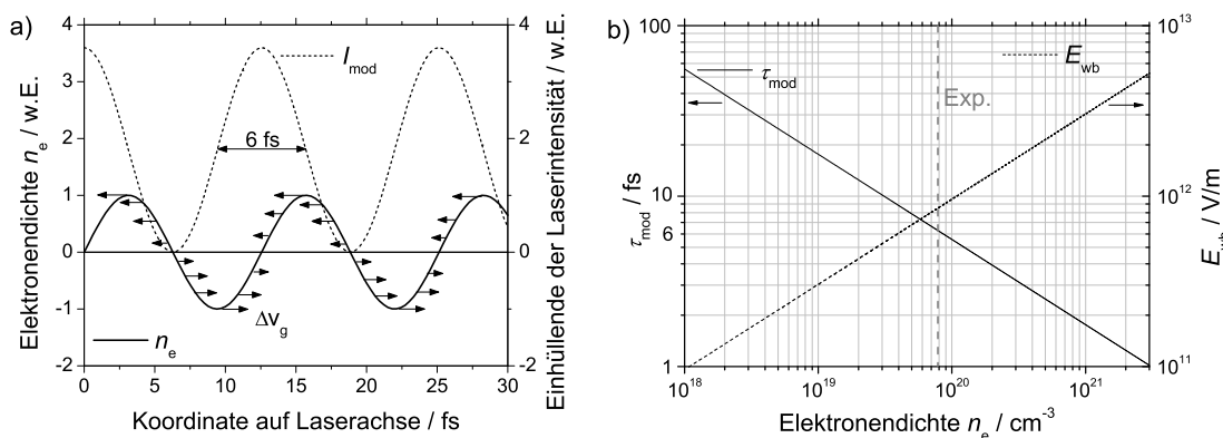
Abbildung 77: a) Selbstmodulation des Laserpulses im Plasma für eine anfängliche Elektronendichte von 8 \cdot 10^{19} \text{ cm}^{-3} führt zur Bildung von Laserfragmenten mit einer Halbwertsbreite von etwa 6 fs (schematische Darstellung, Schnappschuss). b) Die hypothetische Laserpulsfragmentdauer sinkt, und das longitudinale Feld der (klassischen) Plasmawelle E_{wb} steigt mit zunehmender Elektronendichte.
