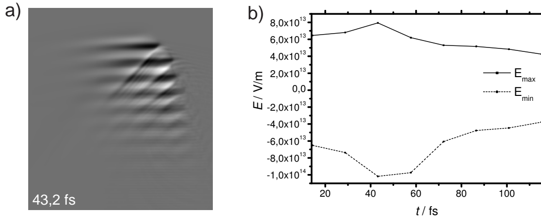
Abbildung 29: a) Vergrößerung des transienten Interferenzfeldes aus Abbildung 28, Bild 3. b) Die aus der PIC-Simulation entnommene Feldüberhöhung ist bei t = 43,2 fs maximal und erreicht einen Wert in der Größenordnung von 10 \text{ TV/m} .
