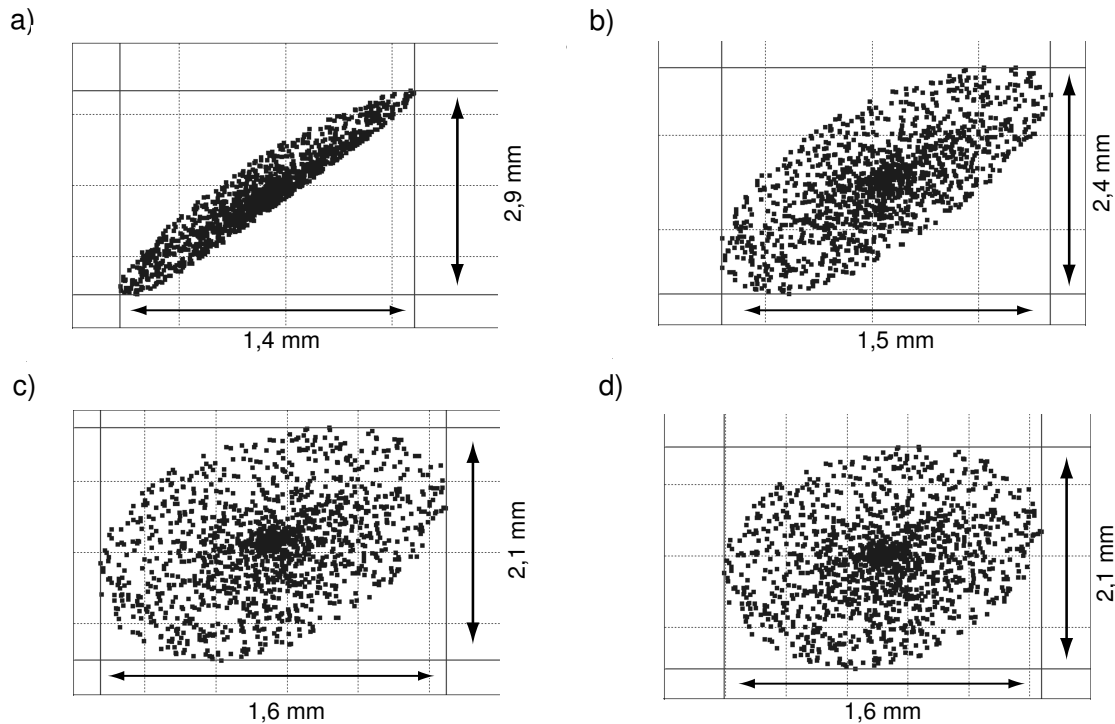
Abbildung 92: Transversale Bunchgröße von Elektronenbunches einer Divergenz von 1 mrad auf der Detektionsebene für a) 100 MeV, b) 200 MeV, c) 500 MeV, d) 1 GeV.
