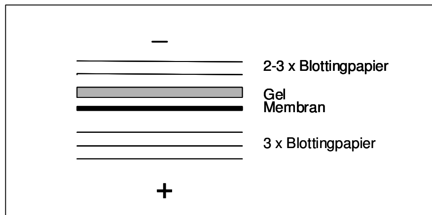
Abb. 2.1: Schematischer Aufbau einer Elektrotransfereinheit für Western Blotting
