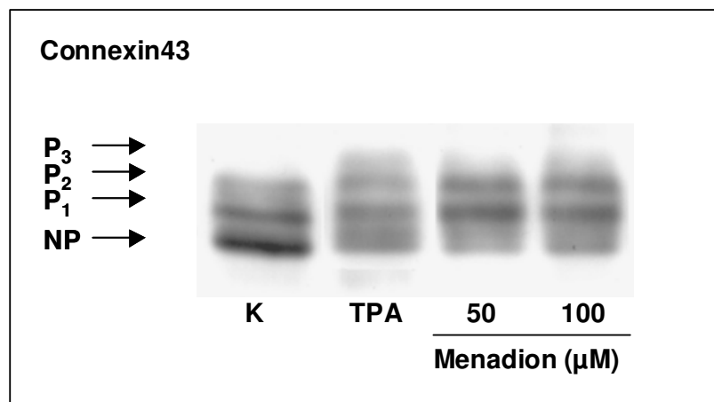
Abb. 3.6: Konzentrationsabhängigkeit der Connexin43-Phosphorylierung durch Menadion. WB-F344 Zellen wurden für 15 min mit 50 und 100 µM Menadion behandelt und lysiert. Die Hyperphosphorylierung durch Menadion wurde mit polyklonalem anti-Connexin43-Antikörper gemessen. Der Vergleich erfolgte durch mit TPA (100 nM) behandelten Zellen (Inkubation, 30 min). Als Kontrolle (K) diente DMSO (0,2%). Die Daten sind repräsentativ für vier unabhängig voneinander durchgeführte Experimente. NP, nicht-phosphorylierte Connexin43-Isoform; P 1 , einfach phosphorylierte, P 2 , doppelt phosphorylierte und P 3 , hyperphosphorylierte Connexin43-Isoform.
