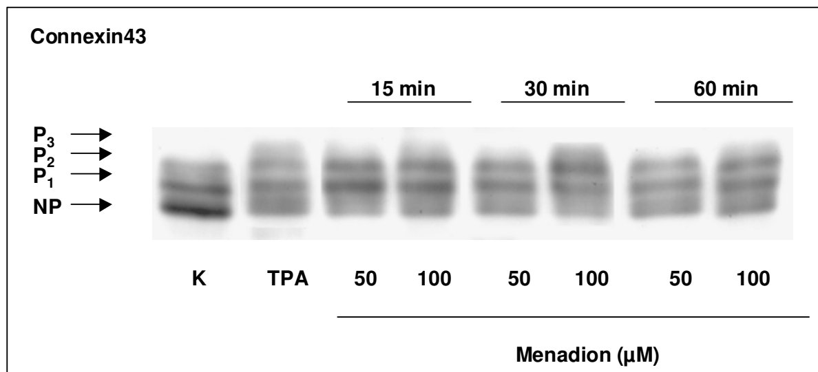
Abb. 3.7: Zeitverlauf der Connexin43-Phosphorylierung durch Menadion. Gezeigt ist ein repräsentativer Western-Blot mit polyklonalem anti-Connexin43-Antikörper. K, Kontrolle (0,2% DMSO). NP, nicht-phosphorylierte Connexin43-Isoform; P_1 , einfach phosphorylierte, P_2 , doppelt phosphorylierte und P_3 , hyperphosphorylierte Connexin43-Isoform.
