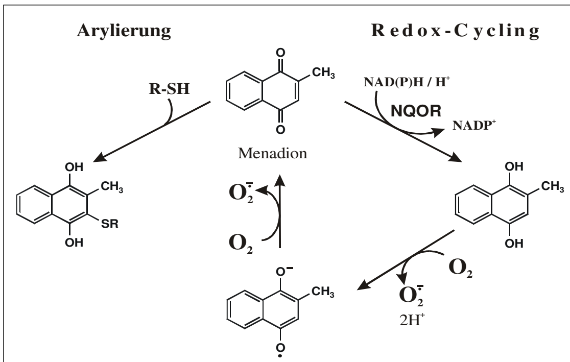
Abb. 1.2: Darstellung des Metabolismus von Menadion. Erläuterungen s. Text.
