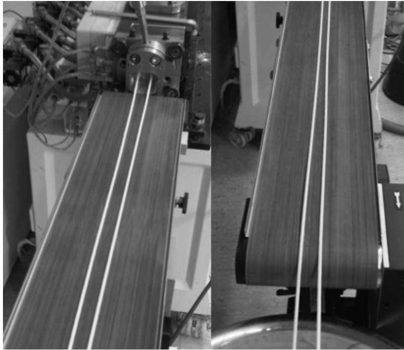
Abb. 40 Kontinuierlichen Schmelzextrusionsprozess mit Poloxamer 188. Transport der Extrudate vom Düsenausgang auf einem Förderband zur Abkühlung und zur zylindrischen Formgebung.
