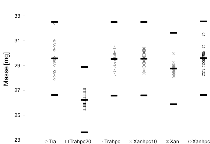
Abb. 23 Einzelmassen mit selbst entwickelter Schneidevorrichtung abgeteilter Arzneiträger (d=3,5 mm, h=2,4 mm, n=20), Markierung von arithmetischem Mittel \pm 10\% (-).
