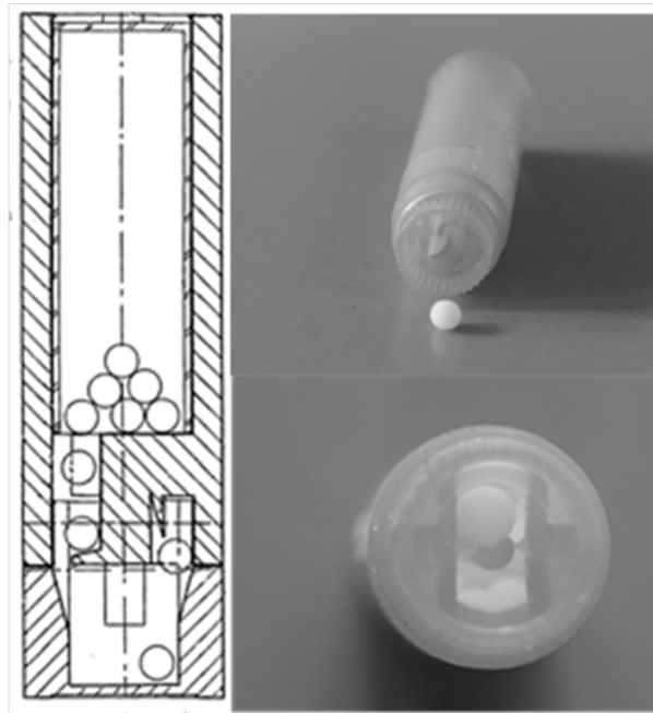
Abb. 9 Technische Zeichnung eines Dosiersystems, (modifiziert nach Laboratoires, Suppo-Steril, 1977 (links)) und Abb. eines Dosiersystems für homöopathische Streukügelchen mit 4 mm Durchmesser (rechts).
