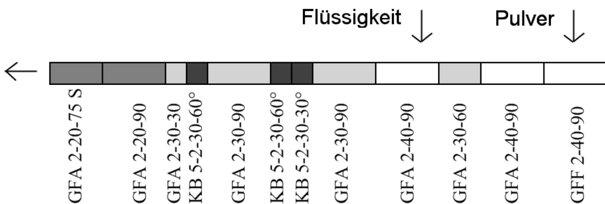
Abb. 52 Schematische Darstellung der Schneckenkonfiguration aus Knetelementen (schwarz) und Förderelementen mit unterschiedlichem Ganglängen (weiß 40 mm, hellgrau 30 mm, dunkelgrau 20 mm).
