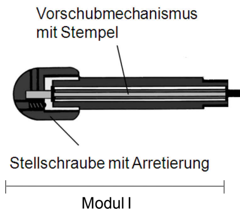
Abb. 14 Technische Zeichnung von Modul I: Vorschubmechanismus mit Stellschraube.
