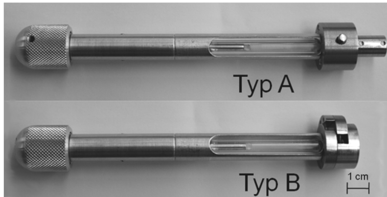
Abb. 17 Prototypen des Dosiersystems in zwei Varianten (Typ A und B), die sich in der Schneidevorrichtung unterscheiden.
