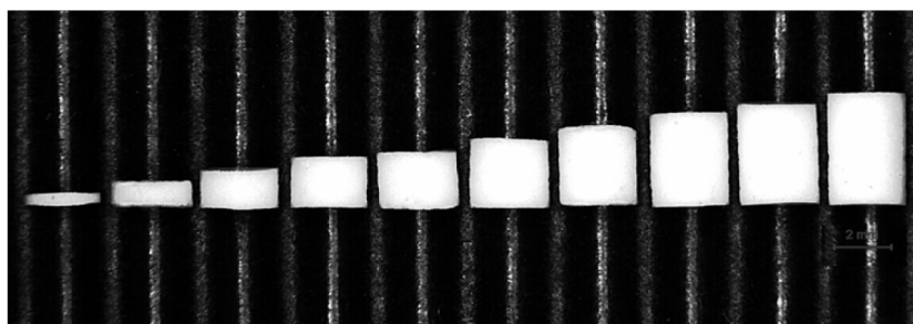
Abb. 32 Zylindrische Arzneiträger der Zubereitung MetoXan25 ( d=2,7\text{ mm} ) mit unterschiedlichen Höhen, dosiert mit dem SDP.
