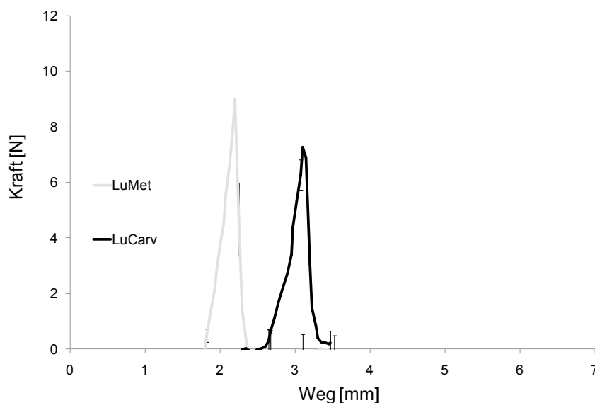
Abb. 45 Kraft-Weg-Diagramm zur Verfolgung des Abteilvorgangs für Schmelzextrudate (d=3,0 mm), MW \pm s, n=10.
