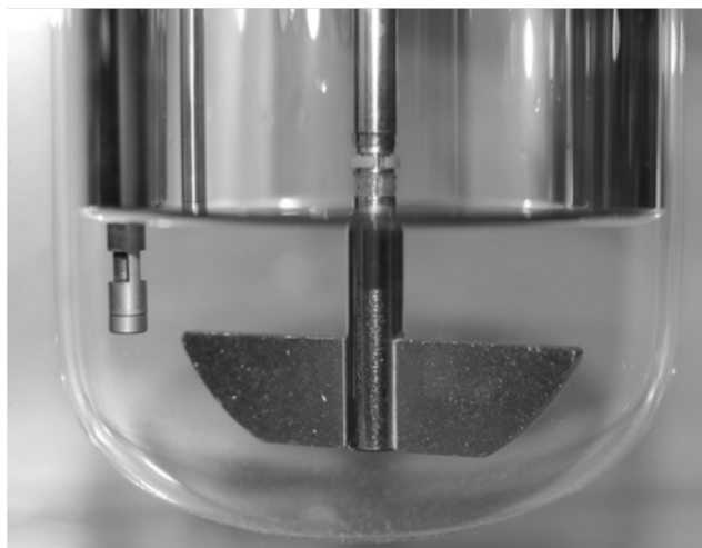
Abb. 53 Faseroptische UV-Tauchsonde im Versuchsaufbau in Freisetzungsgefäß mit Blattrührerapparatur (200 ml Medium).
