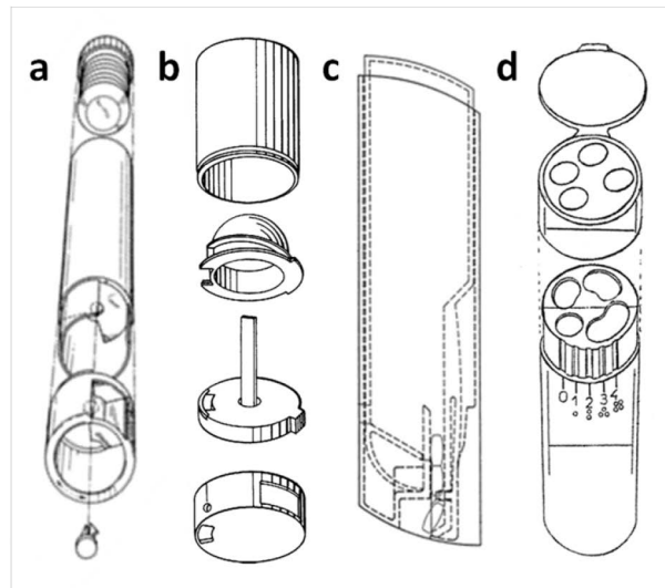
Abb. 10 Technische Zeichnungen von Dosiersystemen, (modifiziert nach Angaben in der Patentliteratur. a: (Schoenefeld, 1980), b: kindergesicherter Dispenser (Uroshevich et al., 1975), c: (Hansen, 1993), d: (Salamé, 1991)).
