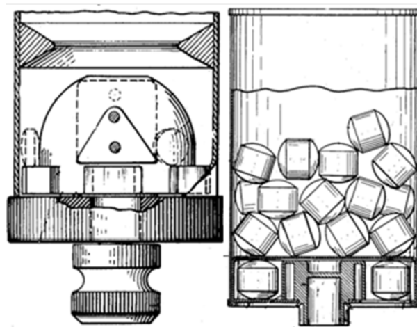
Abb. 8 Technische Zeichnungen von Behältern mit Tabletten, die zur Abgabe einzelner Tabletten geeignet sind, (modifiziert nach Warren, 1940 (links) und Dobkin, 1950 (rechts)).
