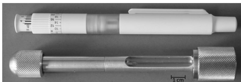
Abb. 18 Prototyp des Solid Dosage Pens (unten) im Größenvergleich zu einem Insulinpen (OptiSet, Sanofi-Aventis).
