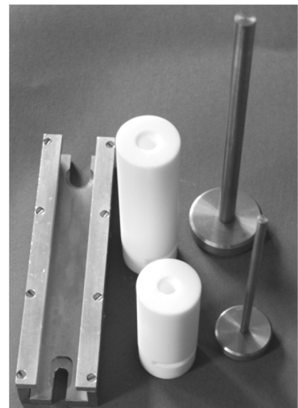
Abb. 51 Neu entwickeltes Werkzeug für die Herstellung zylindrischer Komprimata und die direkte Überführung in ein Packmittel.
