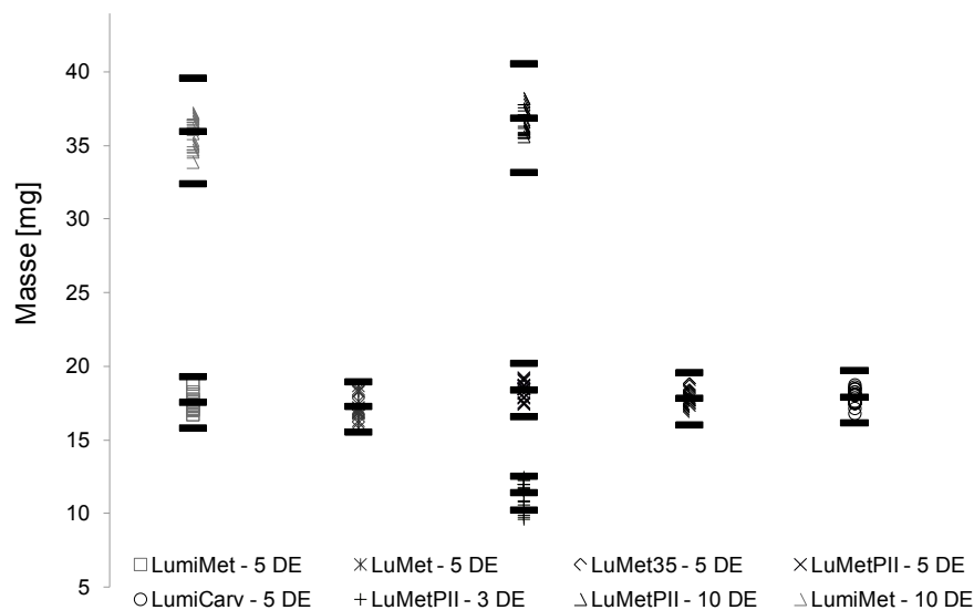
Abb. 46 Einzelmassen mit dem SDP abgeteilter Arzneiträger (d=3,0 mm, 3, 5 und 10 Dosiseinheiten (DE), n=20), Markierung von arithmetischem Mittel \pm 10% (-) nach Ph.Eur. 2.9.27.
