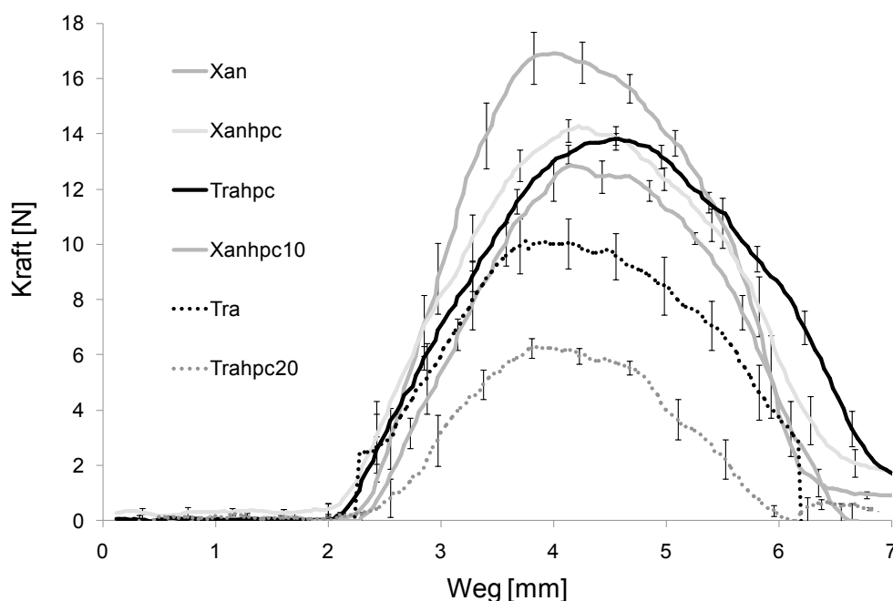
Abb. 22 Kraft-Weg-Diagramm zur Verfolgung des Abteilvorgangs für verschiedene Zubereitungen mit Carvedilol (d=3,5 mm), MW \pm s, n=10.
