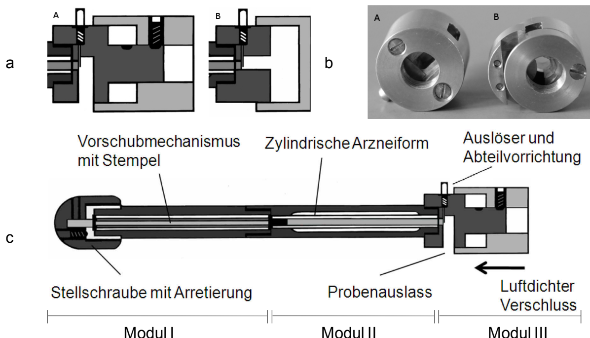
Abb. 16 a: Technische Zeichnung von Modul III in zwei Varianten: Typ A - Arzneiträger fällt nach dem Abteilen durch Probenauslass; Typ B - Arzneiträger liegt während des Abteilens auf und wird dann herausgegeben. b: Klingen in den Prototypen der beiden Varianten. c: Technische Zeichnung des vollständigen Dosiersystems mit Aufsatz Typ A.
