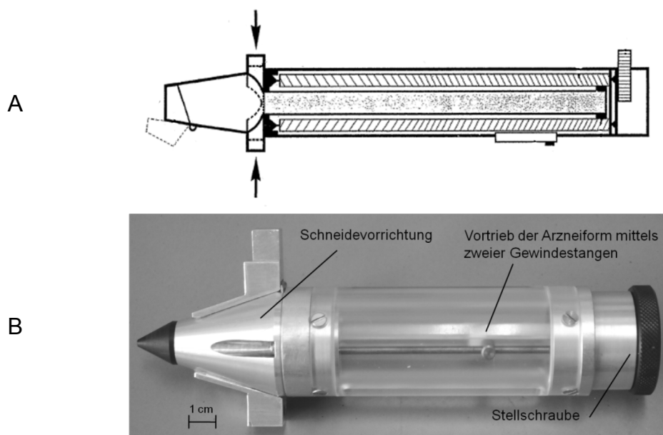
Abb. 13 Technische Zeichnung aus der Patentanmeldung von Schomakers und Grummel (a), selbst gebauter Prototyp nach der Patentanmeldung (b).
