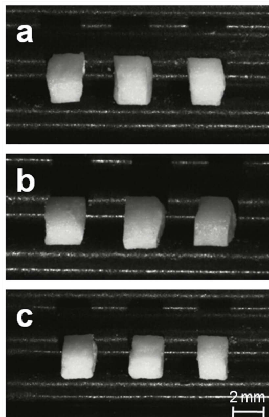
Abb. 47 Mittels SDP abgeteilte Arzneiträger ( d=3 mm, h=2 mm) der Schmelzextrudate verschiedener Zubereitungen. a: LuMet, b: LumiMet und c: LuMetPII.
