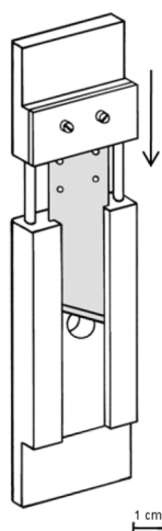
Abb. 55 links: Technische Zeichnung einer neu entwickelten Schneidevorrichtung zur Aufnahme von Kraft-Weg Diagrammen während des Abteilvergangs, rechts: Abbildung in der Versuchsausführung mit waagrecht platziertem Extrudat, d=2,7 mm.
