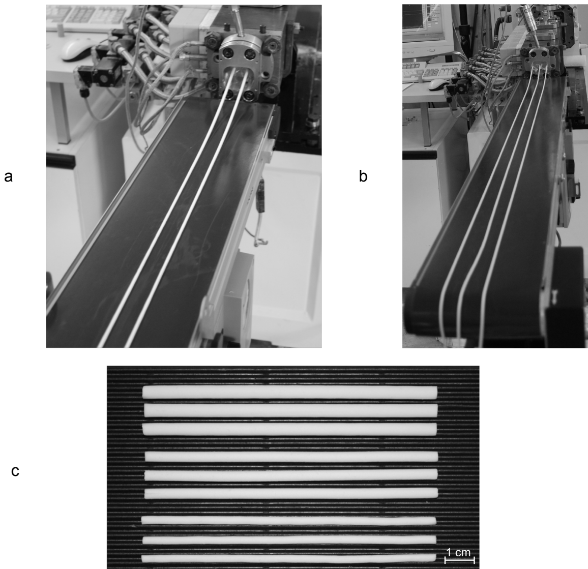
Abb. 21 Kontinuierlicher Feuchtextrusionsprozess mit einem Düsendurchmesser von 4,5 mm (a) und 2,7 mm (b) und Beispiele für geschnittene Extrudate mit einer Länge von 10 cm für alle drei verwendeten Lochdurchmesser in der Düsenplatte (c).
