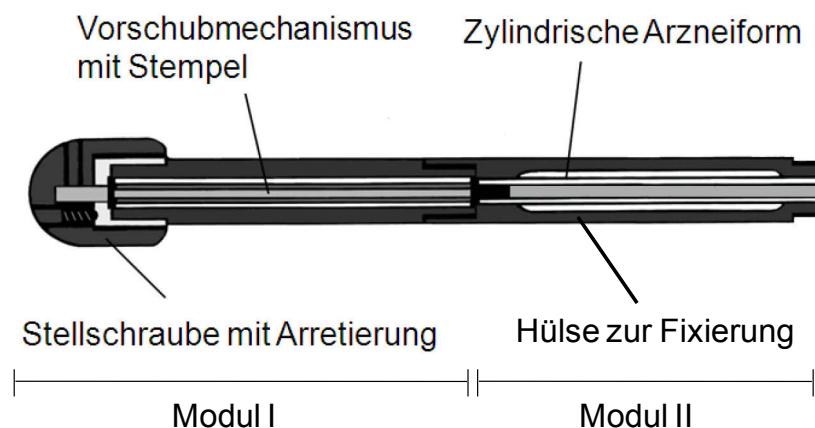
Abb. 15 Technische Zeichnung von Modul II: Fixierung der Arzneiform (verbunden mit Modul I).
