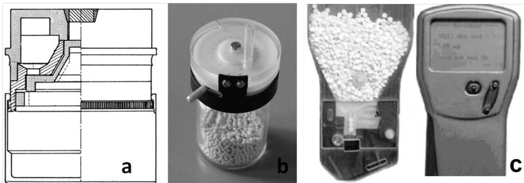
Abb. 11 Dosierer, die mittels einer drehenden Mechanik die Anzahl Untereinheiten auswählen. a: Technische Zeichnung, (modifiziert nach (Schuster, 1988)). b: Prototyp eines Dosierers nach (Breitkreutz und Wazlawik, 2005). c: Elektronisch gesteuertes Dosiersystem zur Abgabe von Minitabletten (modifiziert nach (Bredenberg et al., 2003)).
