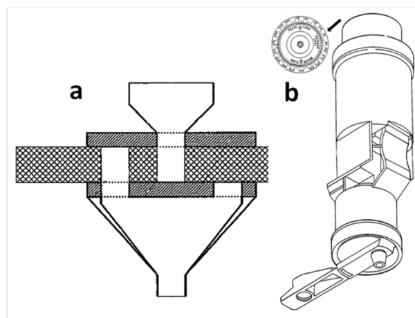
Abb. 6 Technische Zeichnungen zweier Dosierer für festes fließfähiges Material, (modifiziert nach Bauriegel, 2007 (a) und Heimlich, 1984 (b)).
