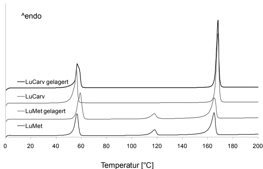
Abb. 49 DSC Thermogramme der Schmelzextrudate LuCarv und LuMet vor und nach 9-monatiger Lagerung unter Stressbedingungen (40°C, 75% rF), jeweils 1. Aufheizkurve, Aufheizrate 10°K/min.
