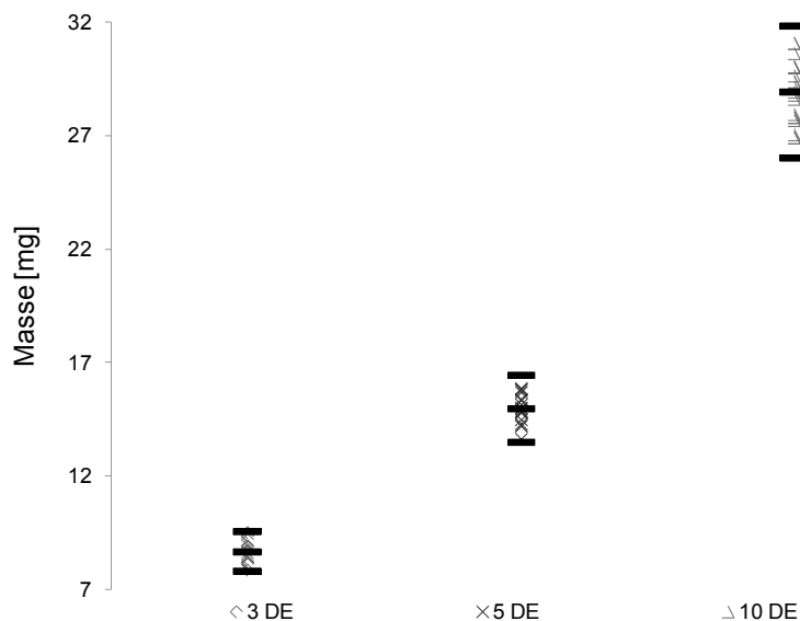
Abb. 38 Einzelmassen mit dem SDP abgeteilter Brause-Arzneiträger (d=3,0 mm, 3, 5 und 10 Dosiseinheiten (DE), n=20), Markierung von arithmetischem Mittel \pm 10\% (-) nach Ph.Eur. 2.9.27.
