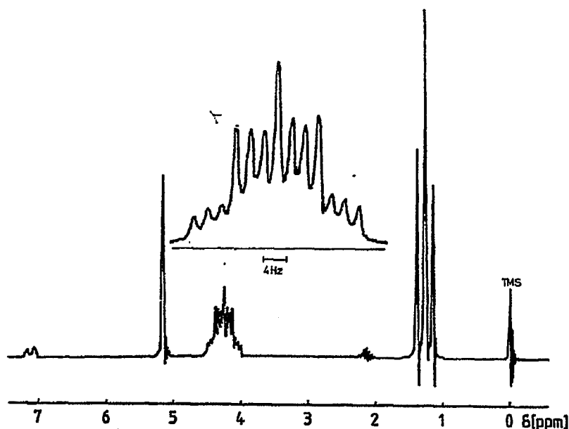
Fig. 1. 60 MHz- ^1\text{H} -NMR Spektrum von I in Toluol- d_8 .
