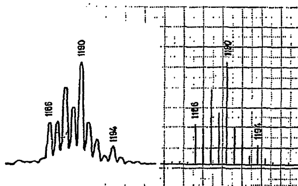
Fig. 2. Beobachtete und berechnete Isotopenverteilung des Molekülions von I.
