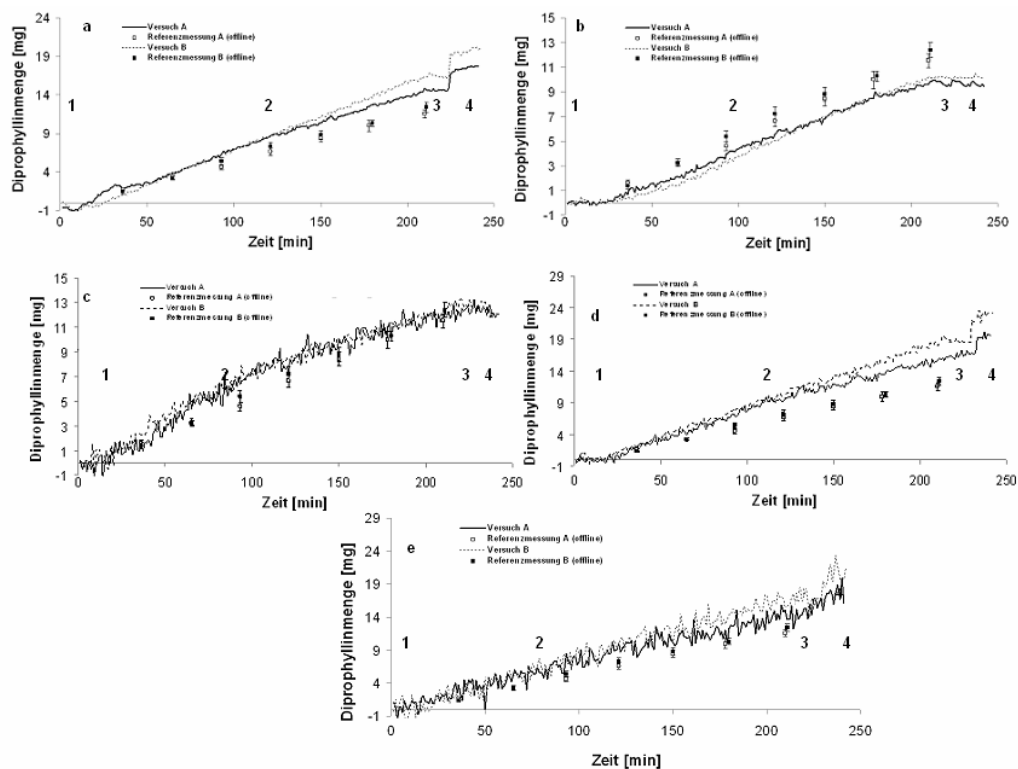
Abbildung 7-8: Vorhersage der aufgetragenen Diprophyllinmenge (mg) anhand der inline Messung in Abhängigkeit von der Datenvorbehandlung ( 500-600\text{ cm}^{-1} ); (a) ohne Vorbehandlung, (b) SNV, (c) MSC, (d) 1. Ableitung, (e) 2. Ableitung; Vergleich mit UV-Referenzwert ( n=9 ; M_w \pm \text{Stabw} ); Prozessabschnitte 1: Aufwärmphase, 2: Coatingphase, 3: Trocknungsphase, 4: Abkühlphase (vgl. Kapitel 3.4.3.2.3)
