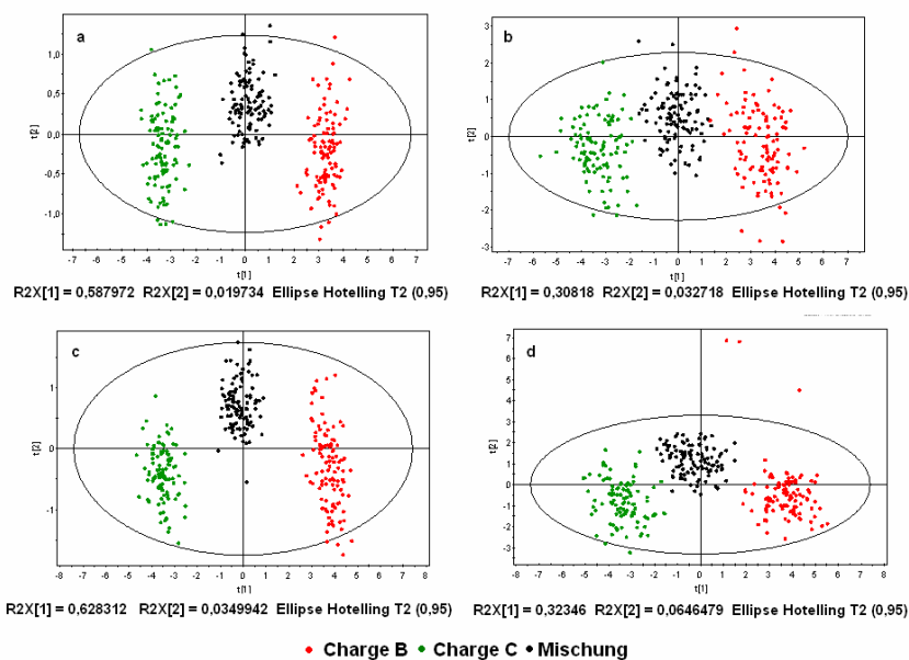
Abbildung 7-15: PCA der Messungen auf der Drehscheibe der reinen Chargen B und C und deren Mischung (alternierende Anordnung; n=105 ; v=0,34 m/s (a) 500 ms (b) 150 ms; v=0,1 m/s, (c) 500 ms (d) 150 ms)(vgl. Kapitel 3.6.2.2)
