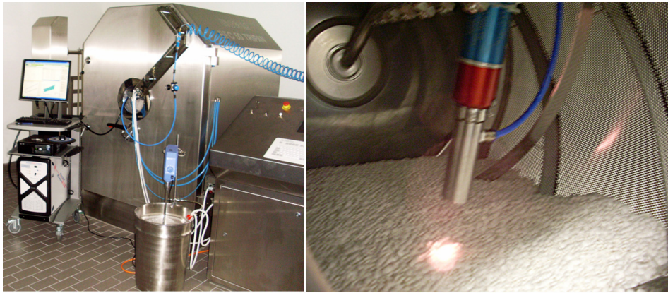
Abbildung 6-5: (a) Versuchsaufbau für die inline Messungen beim BFC 50 Tripan und (b) Befestigung der Ramansonde an der Stange der CIP-Düsen
