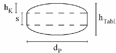
Abbildung 6-13: Abmessungen einer bikonvexen runden Tablette [nach [119]]
