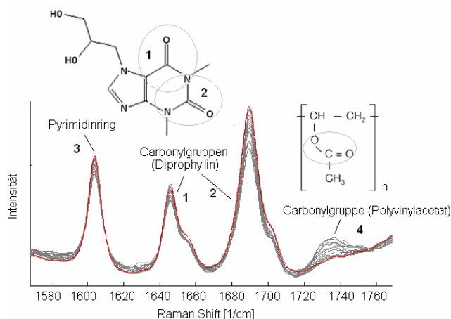
Abbildung 3-60: Intensität in Abhängigkeit von der Coatingzeit im Wellenzahlbereich 1550\text{-}1810\text{ cm}^{-1}
