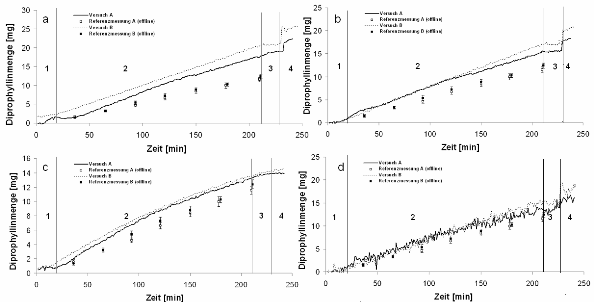
Abbildung 3-36: Vorhersage der aufgetragenen Diprophyllinmenge (mg) anhand der inline Messung in Abhängigkeit von der Datenvorbehandlung (1200-1400 \text{cm}^{-1} ): (a) ohne Vorbehandlung, (b) 1. Ableitung, (c) MSC, (d) 2. Ableitung; Vergleich mit UV-Referenzwert (n=9; M_w \pm \text{Stabw} ); Prozessabschnitte 1: Aufwärmphase, 2: Coatingphase, 3: Trocknungsphase, 4: Abkühlphase
