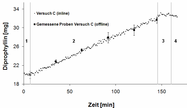
Abbildung 3-25: Vorhersage der Diprophyllinmenge (mg) anhand der inline Messung; Vergleich mit UV-Referenzwert ( n=9 ; M_w \pm \text{Stabw} ); Prozessabschnitte 1: Aufwärmphase, 2: Coatingphase, 3: Trocknungsphase, 4: Abkühlphase
