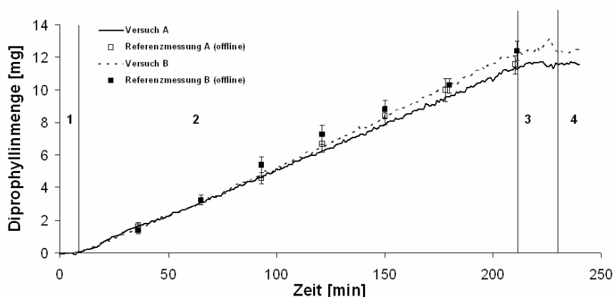
Abbildung 3-38: Vorhersage der aufgetragenen Diprophyllinmenge (mg) anhand der inline Messung mit Hilfe des erstellten MCR-Modells; Vergleich mit UV-Referenzwert (n=9; M_w \pm \text{Stabw} ); Prozessabschnitte 1: Aufwärmphase, 2: Coatingphase, 3: Trocknungsphase, 4: Abkühlphase
