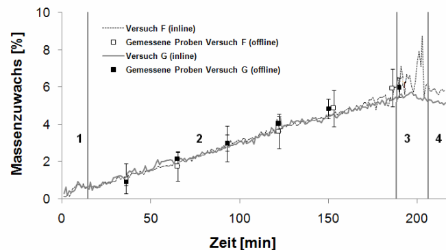
Abbildung 3-30: Vorhersage des Massenzuwachses (%) anhand der inline Messung; Vergleich mit Gravimetrie-Referenzwert ( n=30 ; M_w \pm \text{Stabw} ); Prozessabschnitte 1: Aufwärmphase, 2: Coatingphase, 3: Trocknungsphase, 4: Abkühlphase
