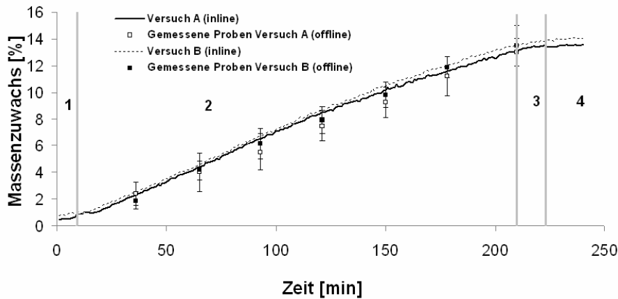
Abbildung 3-20: Vorhersage des Massenzuwachses (%) anhand der inline Messung; Vergleich mit Gravimetrie-Referenzwert (n=30; Mw ± Stabw); Prozessabschnitte 1: Aufwärmphase, 2: Coatingphase, 3: Trocknungsphase, 4: Abkühlphase.
