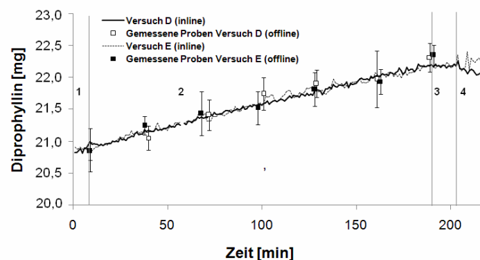
Abbildung 3-29: Vorhersage der Diprophyllinmenge (mg) anhand der inline Messung; Vergleich mit UV-Referenzwert ( n=9 ; M_w \pm \text{Stabw} ); Prozessabschnitte 1: Aufwärmphase, 2: Coatingphase, 3: Trocknungsphase, 4: Abkühlphase
