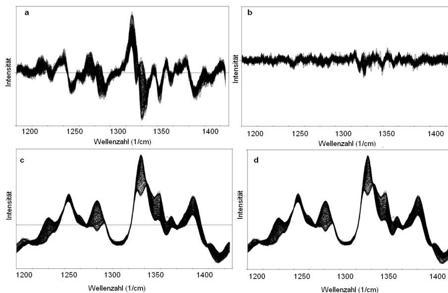
Abbildung 7-7: Anhand der inline Messung erhaltene Ramanspektren in Abhängigkeit von der Datenvorbehandlung ; (a) 1. Ableitung, (b) 2. Ableitung, (c) SNV und (d) MSC (vgl. Kapitel 3.4.3.2.2)
