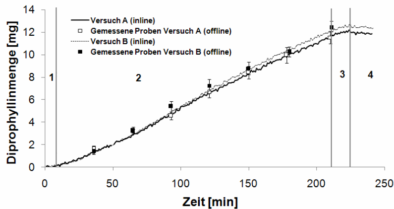
Abbildung 3-17: Vorhersage der aufgetragenen Diprophyllinmenge (mg) anhand der inline Messung; Vergleich mit UV-Referenzwert (n=9; M_w \pm \text{Stabw} ); Prozessabschnitte 1: Aufwärmphase, 2: Coatingphase, 3: Trocknungsphase, 4: Abkühlphase.
