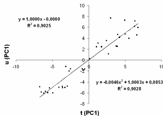
Abbildung 3-68: u-/t- Score Diagramm der 1. Hauptkomponente nach erfolgter Transformation der X-Variablen
