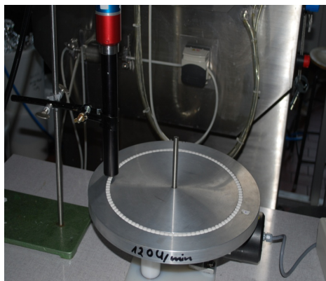
Abbildung 6-9: Versuchsaufbau für die Untersuchung der Coating Uniformity (vgl. Kapitel 3.6.2)
