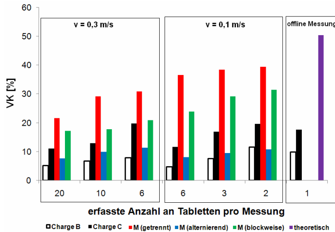
Abbildung 3-56: VK der ermittelten Diprophyllinmenge ( n=105 ) der reinen Chargen und der Mischungen in Abhängigkeit von der erfassten Anzahl an Tabletten pro Messung im Vergleich mit dem anhand der offline Messung theoretisch zu erwartenden VK
